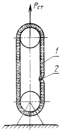
1 -образец покрытия; 2 -шов Черт.5
