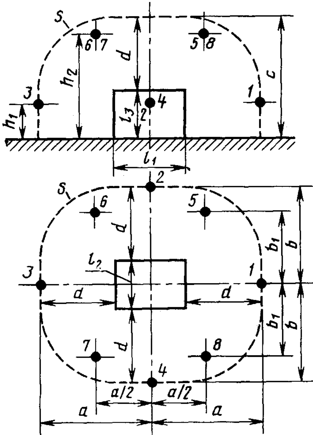
S - измерительная поверхность; 1-8 - точки измерения; l_1, l_2, l_3 - размеры огибающего источника шума параллелепипеда; d - измерительное расстояние; a, b, c - характеристические размеры измерительной поверхности
