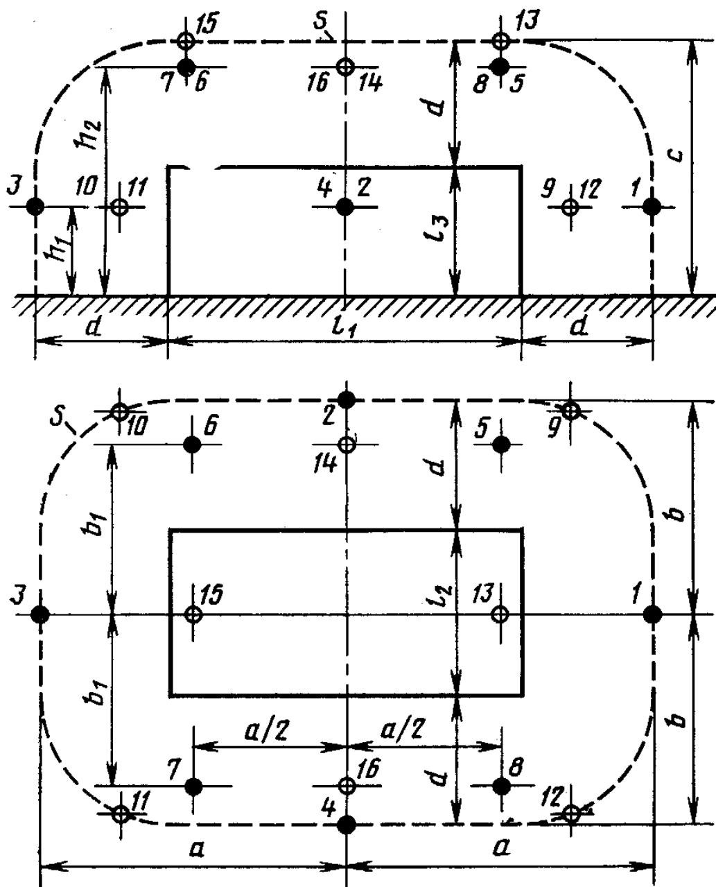
S - измерительная поверхность; 1-8 - точки измерения; 9-16 - дополнительные точки измерения; l_1, l_2, l_3 - размеры огибающего источника шума параллелепипеда; d - измерительное расстояние; a, b, c - характеристические размеры измерительной поверхности
