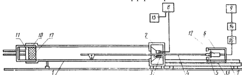
Блок-схема интерферометра
