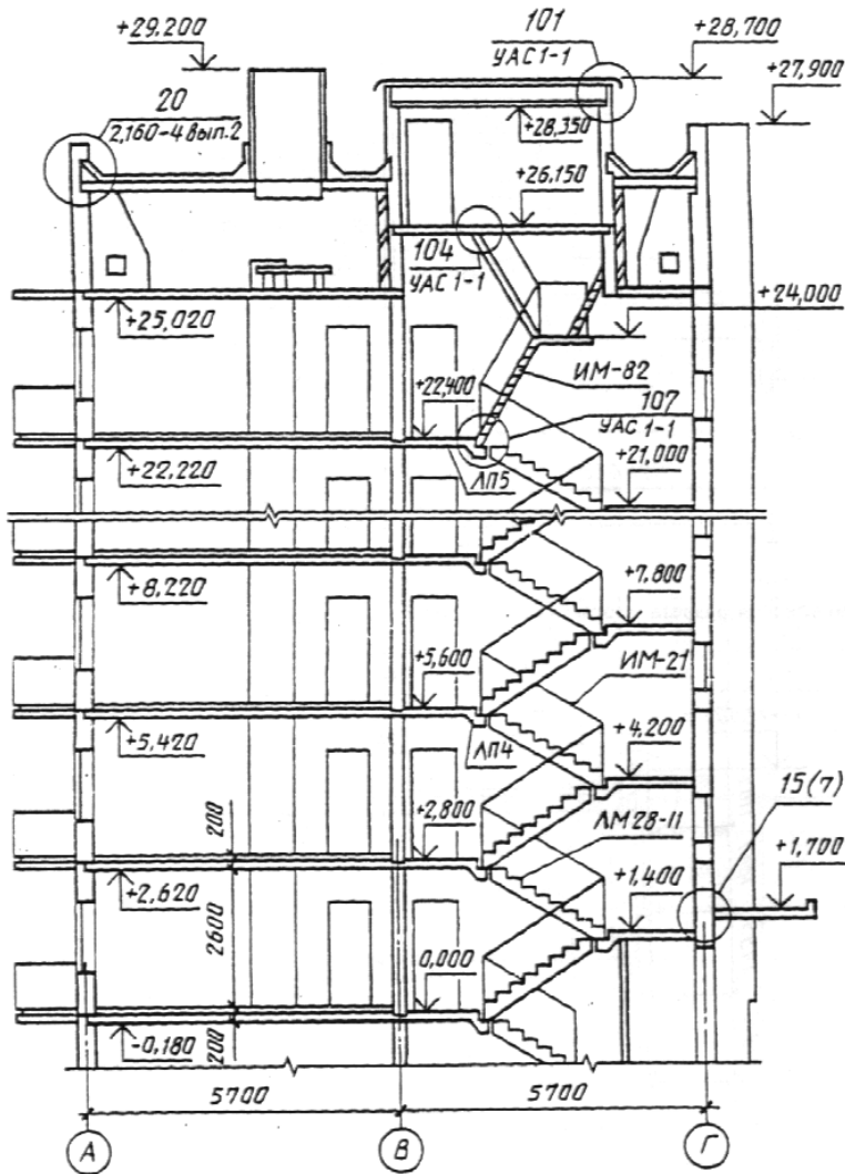
Разрез 1-1
