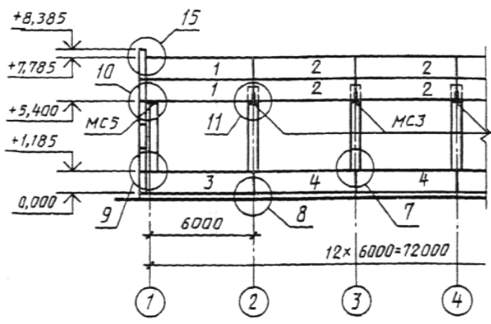
Схема расположения панелей стен
