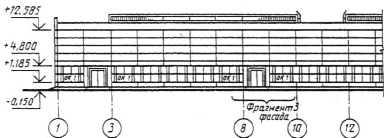
Фрагмент 3 фасада
