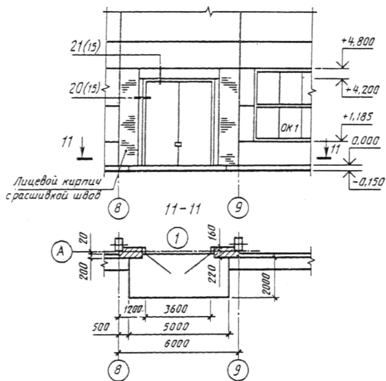
Фрагмент 3 фасада
