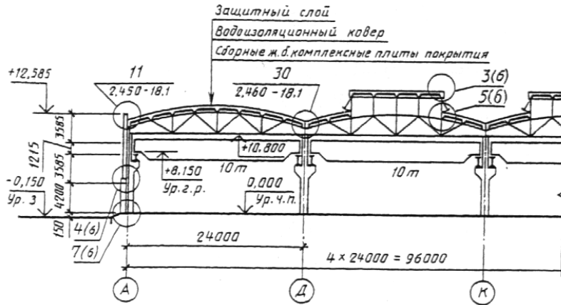
Разрез 1-1
