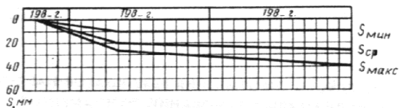
График развития перемещений
