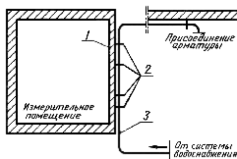
Схема испытательного стенда
