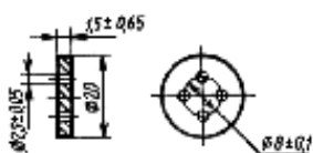
а) диск с четырьмя отверстиями
