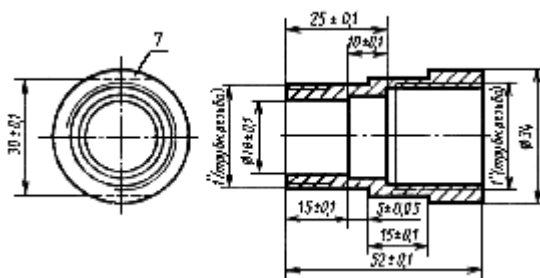
г) сборочный чертеж
