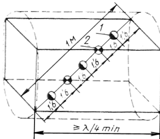
1 - основные измерительные точки; 2 - дополнительные измерительные точки Черт. 8
