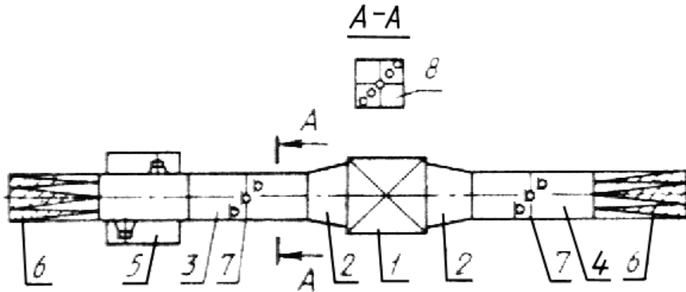
1 - испытываемый глушитель шума; 2 - конфузор или диффузор; 3 - входной измерительный воздуховод; 4 - выходной измерительный воздуховод; 5 - набор громкоговорителей; 6 - концевое поглощающее устройство; 7 - измерительная плоскость; 8 - размещение измерительных точек Черт. 7
