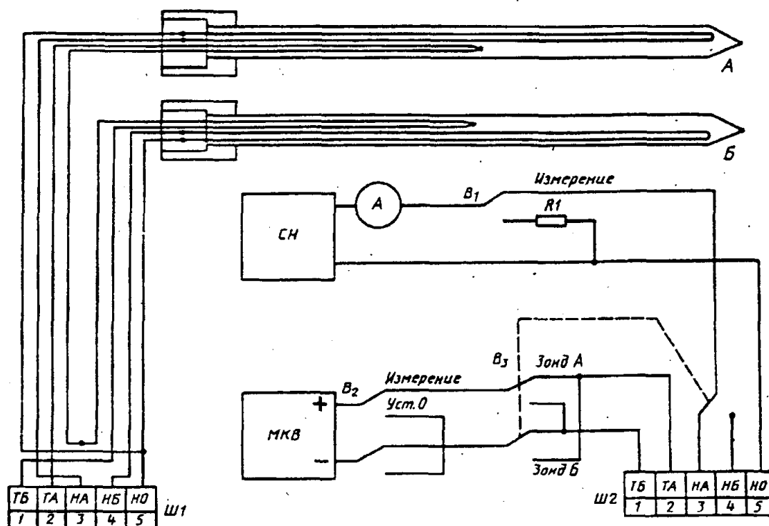
Рисунок 1 — Устройство зонда и электрическая схема соединения приборов
