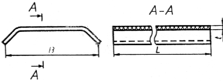
Рисунок 5 - Лотковая деталь
