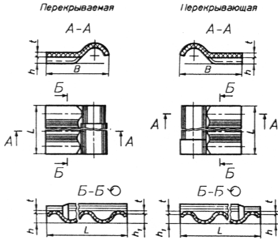
Рисунок 2 - Коньковые детали
