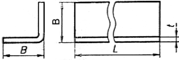
Рисунок 4 - Равнобокая угловая деталь
