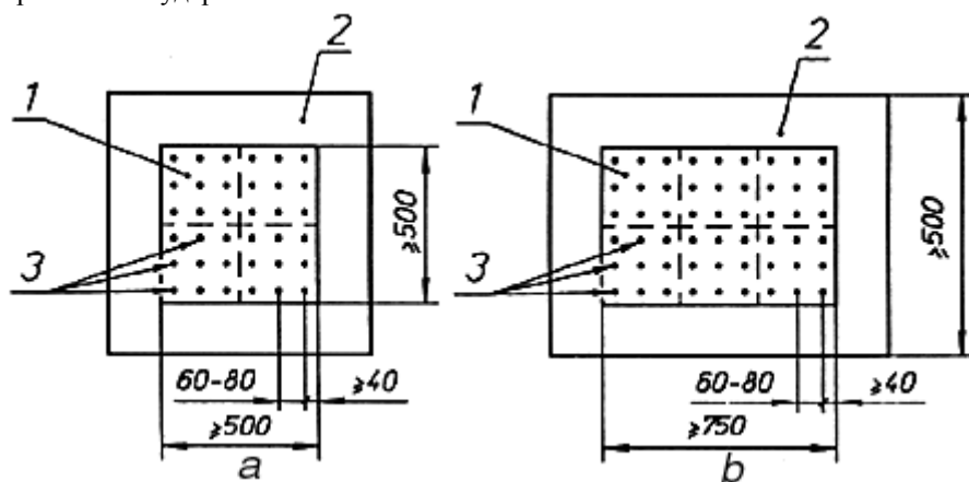
1 - опытный участок; 2 - обрамляющий бортик; 3 - точки приложения ударов
