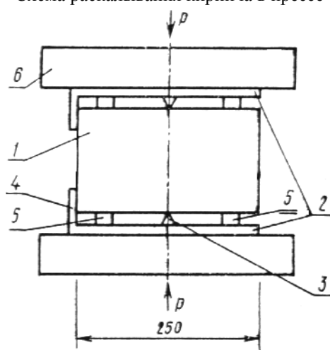
Схема раскалывания кирпича в прессе
