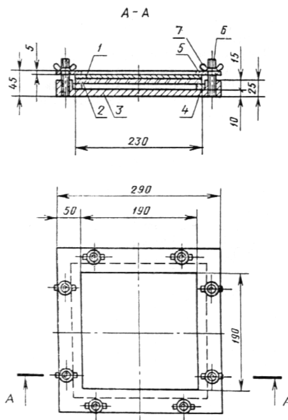
1 — образец; 2 — плита древесностружечная; 3 — основание металлическое; 4 — нижняя рамка; 5 — рамка прижимная стальная; 6 — болт стальной; 7 — гайка-барашек Черт. 2
