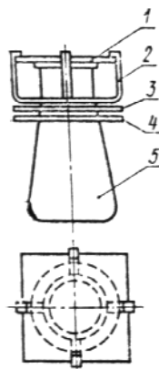
1 — образец; 2 — поддерживающее устройство; 3 — кольцо асбестовое; 4 — кольцо алюминиевое; 5 — колба.
