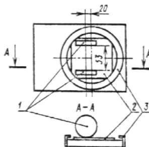
1 — истирающие диски; 2 — образец; 3 — зажимное кольцо.
