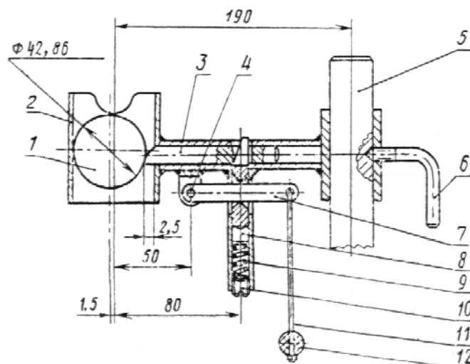
1 — шарик; 2 — кронштейн; 3 — плунжер; 4 — ось; 5 — штанга; 6 — фиксатор; 7 — коромысло; 8 — клин; 9 — пружина; 10 — пробка; 11 — тросик; 12 — рукоятка Черт. 3
