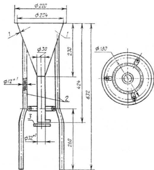
1 — воронка; 2 — опоры; 3 — заслонка
