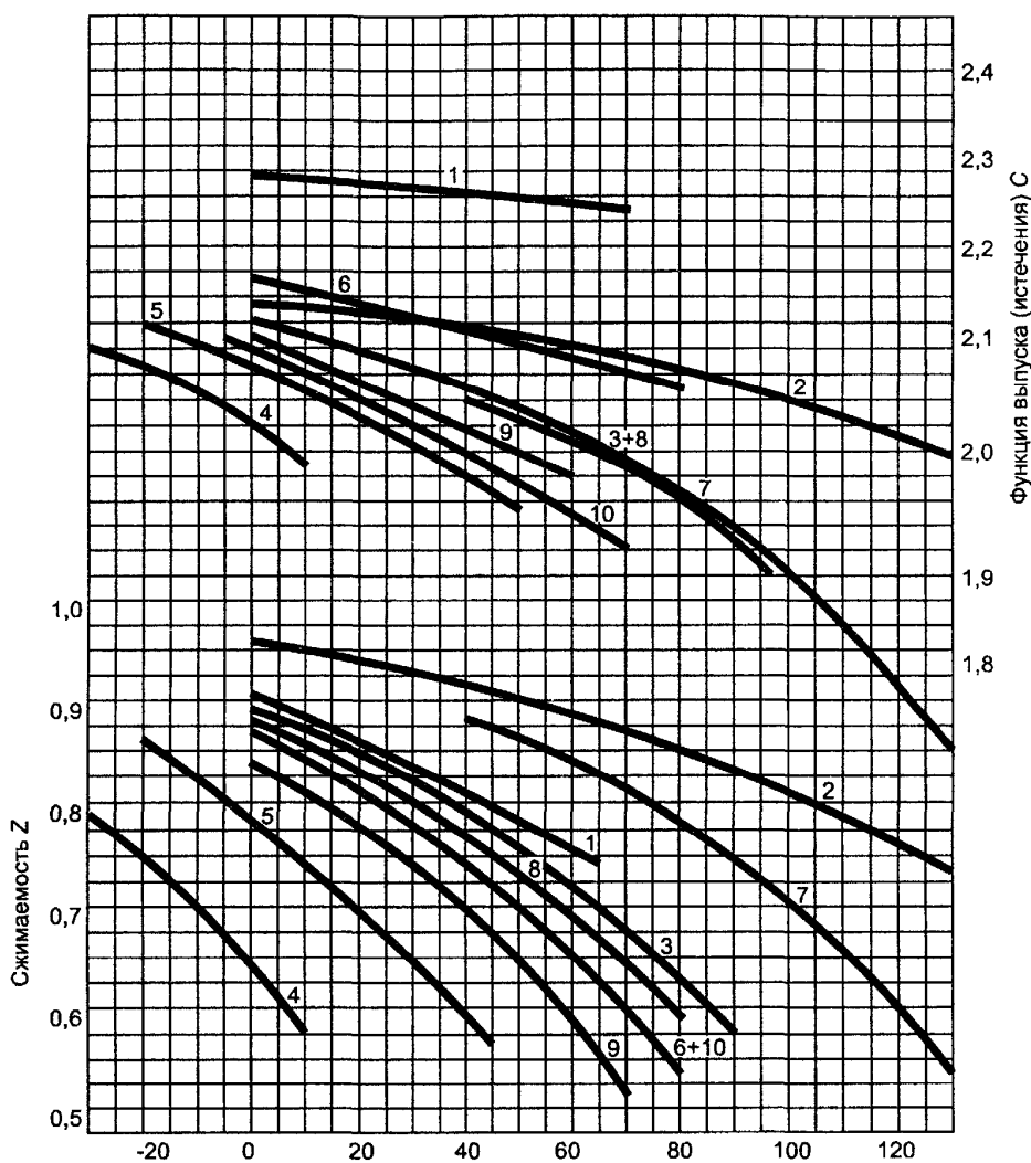
Температура насыщения в камере давления, °С 1-R717; 2-R11; 3-R12; 4-R13; 5-R13B1; 6-R22; 7-R114; 8—R500; 9-R502; 10- пропан
