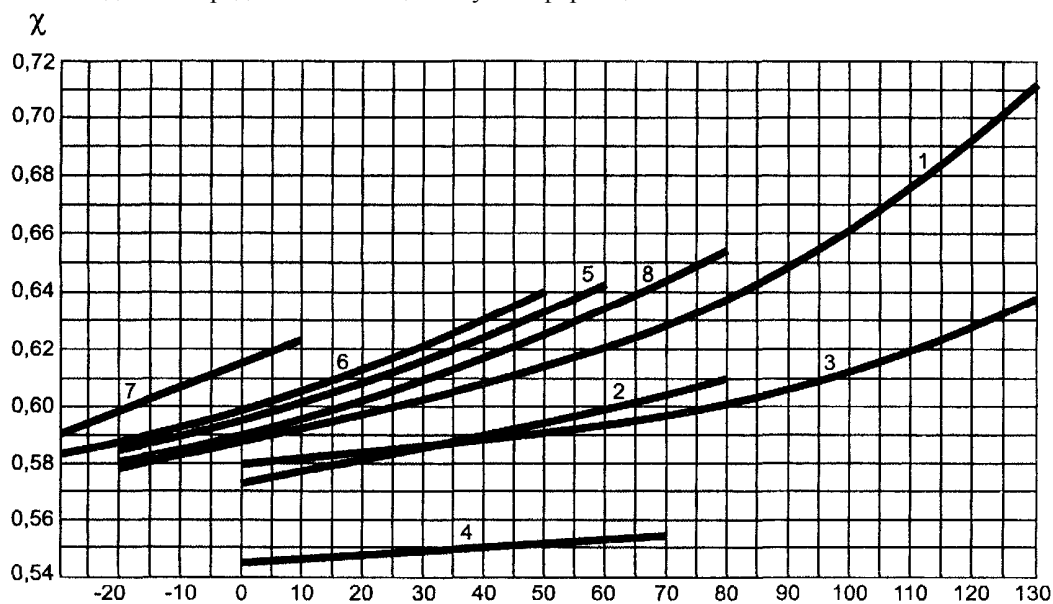
Температура насыщения в камере давления, С 1-R12,R14, R500; 2-R22; 3-R11; 4-R717; 5-R502; 6-R13B1; 7-R13; 8-пропан Рисунок Б.3 — Значение коэффициента \chi для критического давления потока.
