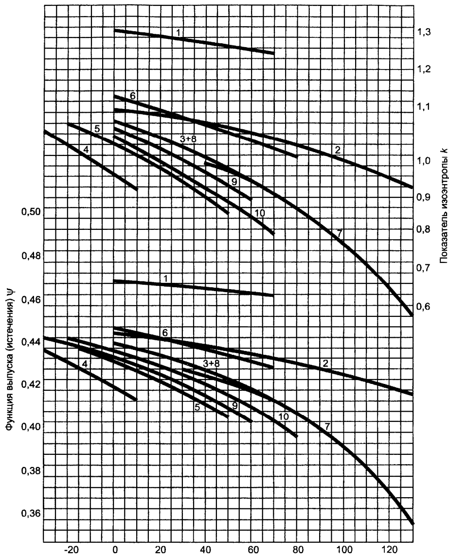
Температура насыщения в камерах давления, °С 1-R717; 2-R11; 3-R12; 4-R13; 5-R13B1; 6-R22; 7-R114; 8-R500; 9-R502; 10 -пропан
