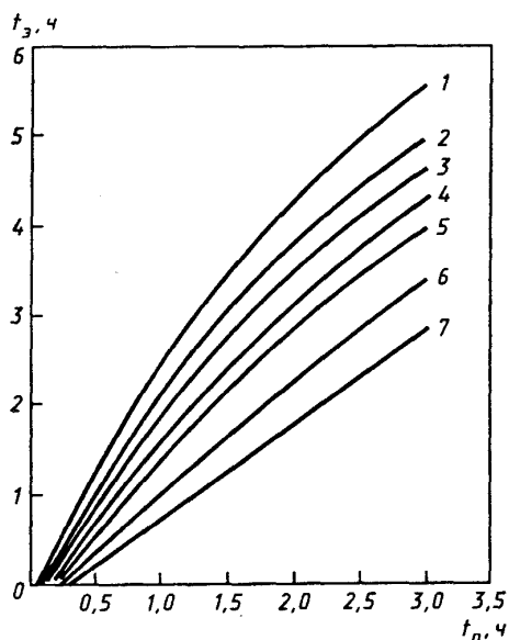
Рисунок Л.7 — Зависимость эквивалентной продолжительности пожара t_3 от характерной продолжительности пожара t_n для огнезащищенных металлических и железобетонных конструкций перекрытия
