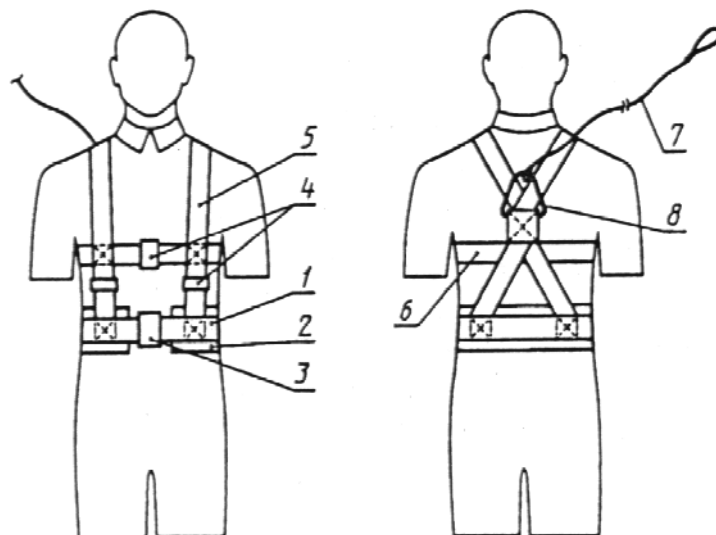
Рисунок 4 — Лямочный пояс, тип Г
