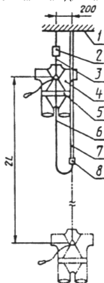
Рисунок 10 — Схема испытания лямочных поясов типов В, Д и Е динамической нагрузкой 1 — жесткая опора; 2 — сбрасыватель; 3 — соединительное устройство; 4 — манекен; 5 — пояс лямочный; 6 — строп; 7 — штанга; 8 — серьга штанги L — максимальная длина стропа.
