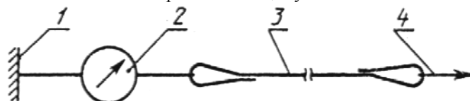
Рисунок 8 — Схема испытания элементов пояса статической нагрузкой 1 — жесткая опора; 2 — измеритель усилия; 3 — строп или другой элемент пояса; 4 — растягивающее усилие
