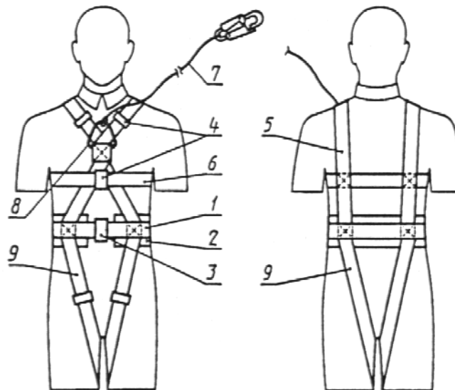
Рисунок 6 — Лямочный пояс, тип Е
