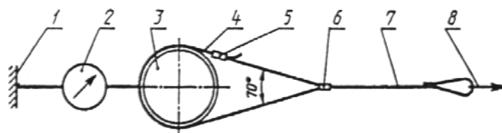
Рисунок 7 — Схема испытания пояса в целом статической нагрузкой 1 — жесткая опора; 2 — измеритель усилия; 3 — цилиндр диаметром 300 мм; 4 — пояс; 5 — пружина; 6 — боковое кольцо пояса; 7 — строп; 8 — растягивающее усилие
