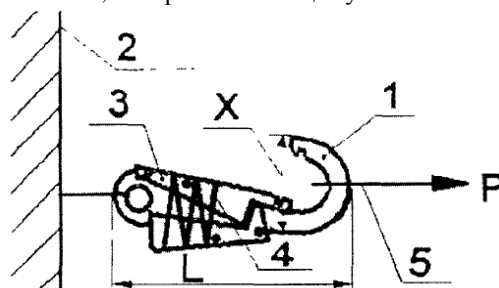
Рисунок 8а - Схема испытания карабина статической нагрузкой 1 - основной крюк карабина; 2 - неподвижная опора; 3 - внутренняя рукоятка карабина; 4 - проволока диаметром 1 - 1,5 мм для закрепления рукоятки в указанном положении; 5 - растягивающее усилие ( 500 \pm 1 кгс); X - расстояние между наружной поверхностью носка крюка карабина и наружной поверхностью тыльной стороны крюка карабина; L - длина карабина, измеренная по оси приложения нагрузки P
