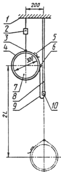
Рисунок 9 — Схема испытания безлямочных поясов типов А и Б динамической нагрузкой 1 — жесткая опора; 2 — сбрасыватель; 3 — соединительное устройство; 4 — пояс безлямочный; 5 — пряжка; 6 — боковое кольцо; 7 — манекен (мешок с песком); 8 — штанга; 9 — строп; 10 — серьга штанги; L — максимальная длина стропа
