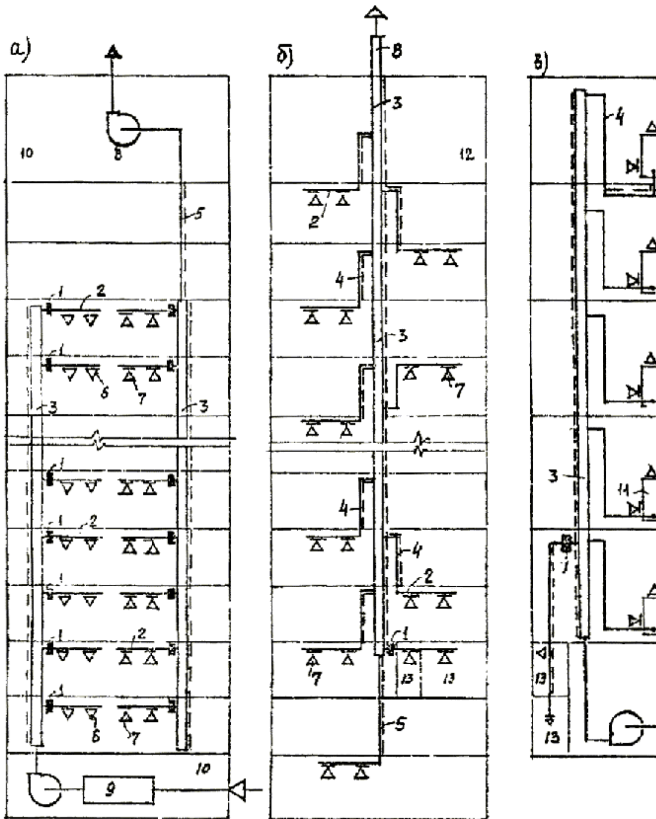
Рис. 1. Схемы воздуховодов с вертикальными коллекторами.
