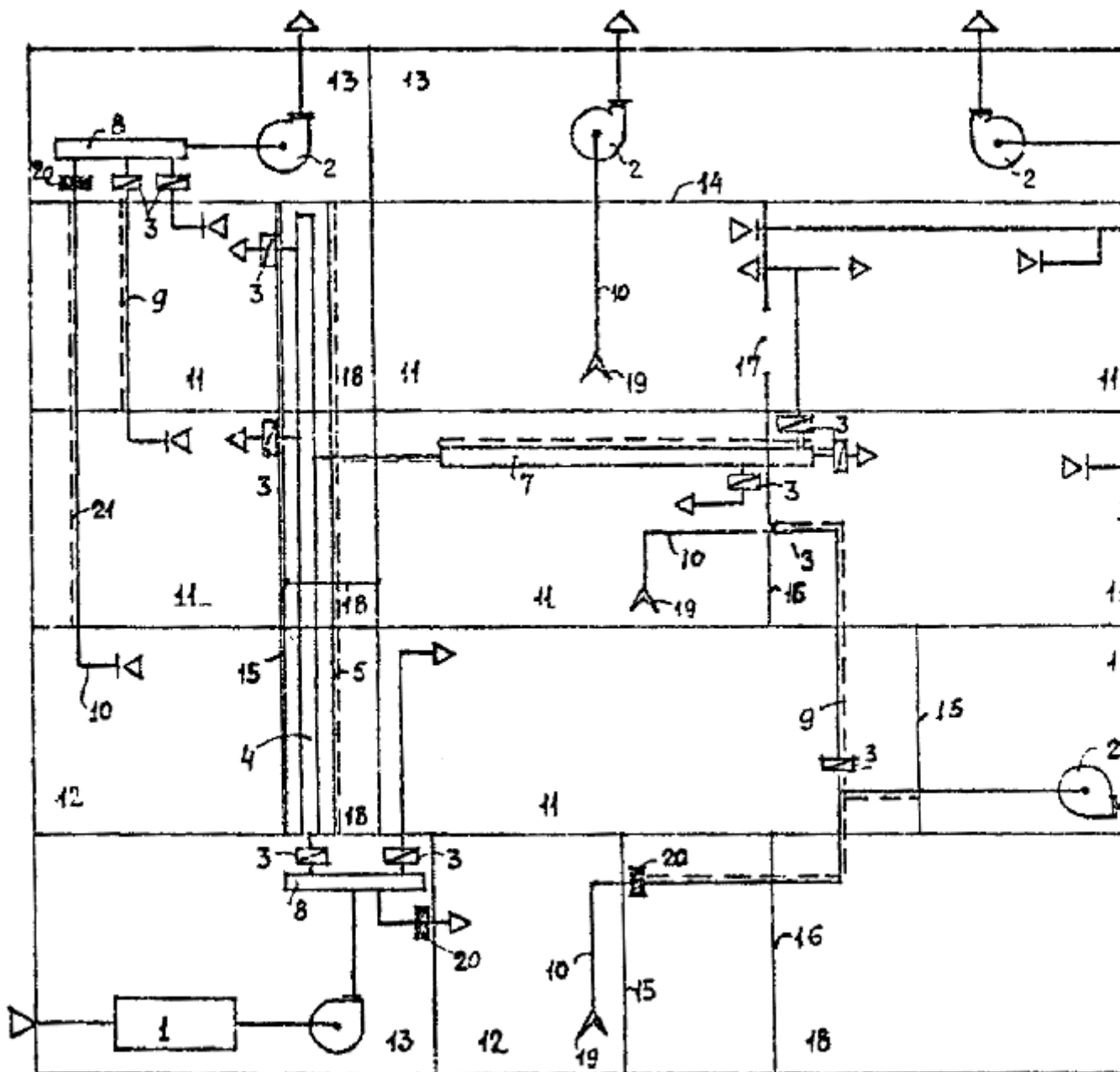
Рис. 4. Схемы воздухопроводов для помещений категории А, Б или В.
