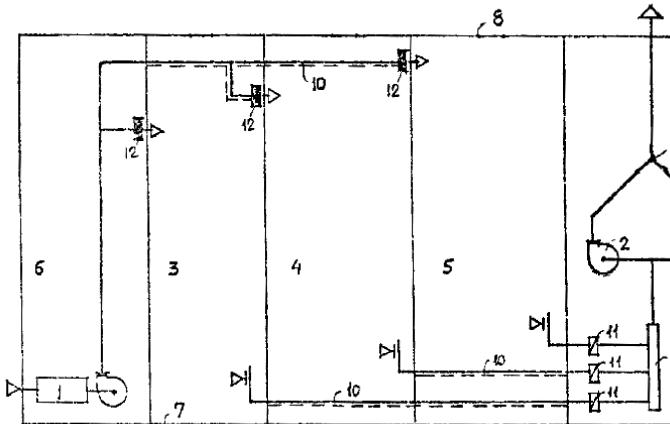
Рис. 5 Схемы воздуховодов для изолированных производственных помещений категорий А, Б или В по п. 4.25 в.
