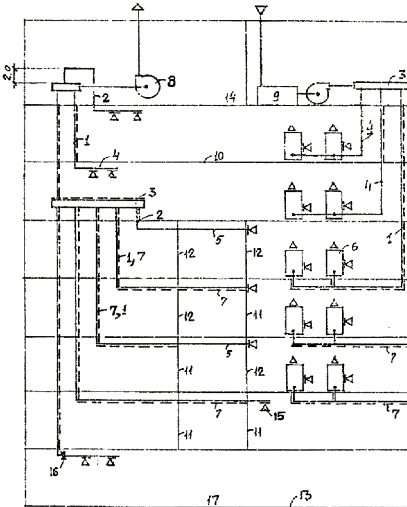
Рис. 2. Схемы воздуховодов с горизонтальными коллекторами.
