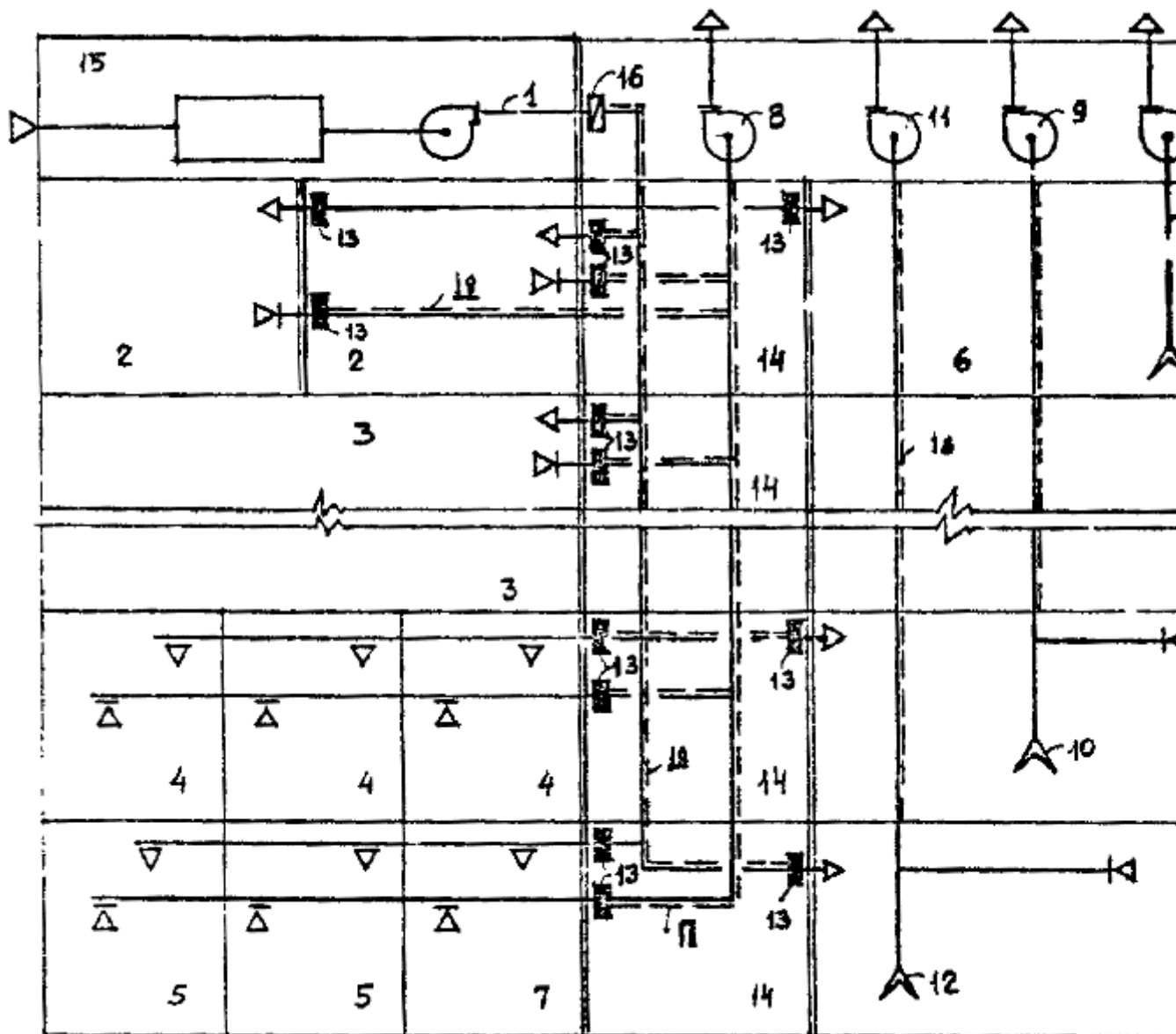
Рис. 7. Схемы воздуховодов для лабораторных помещений.
