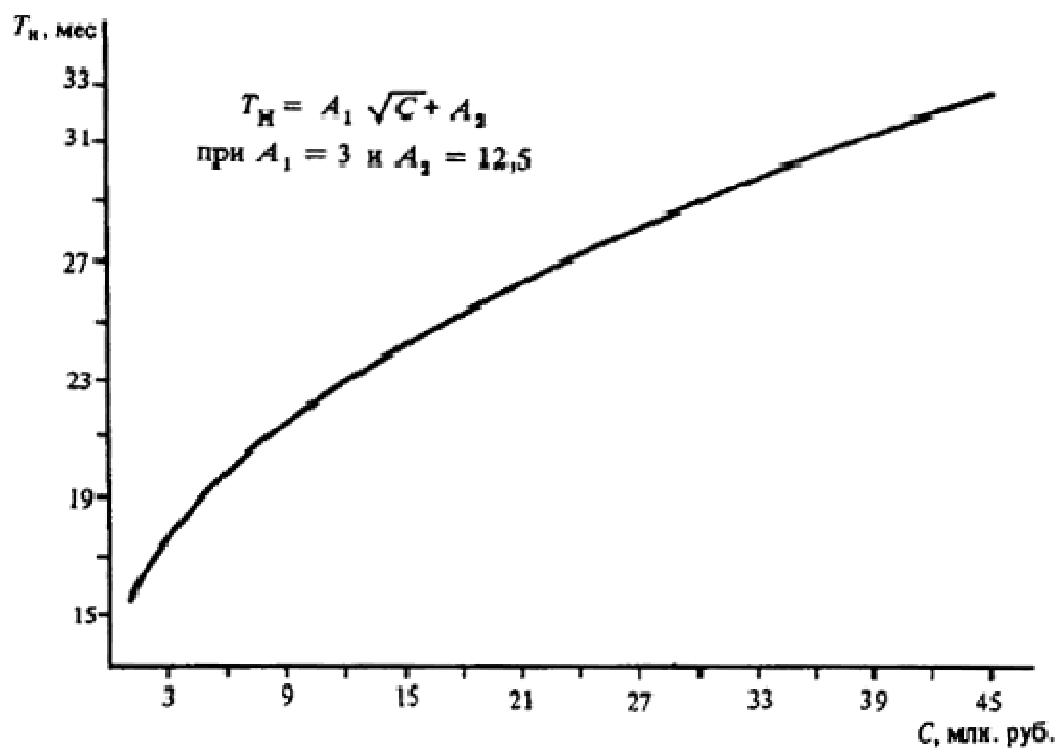
Черт. 55. Определение T_n объектов воздушного транспорта
