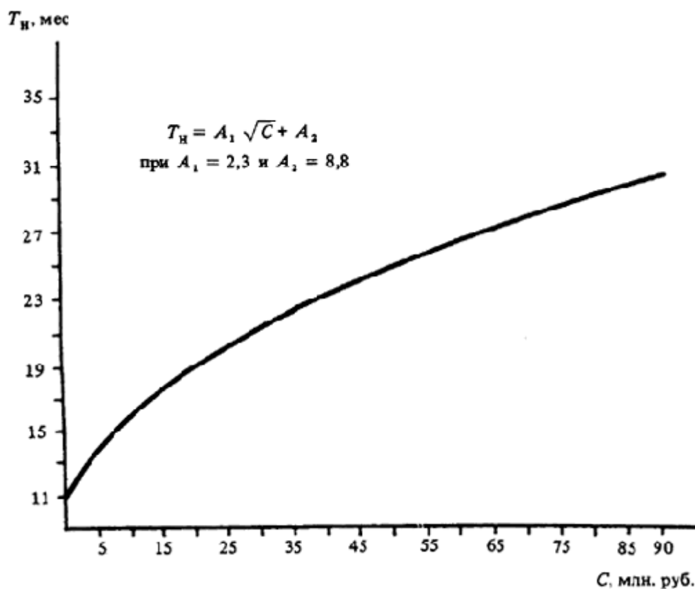
Черт. 9. Определение T_n сталеплавильного, ферросплавного и огнеупорного производства
