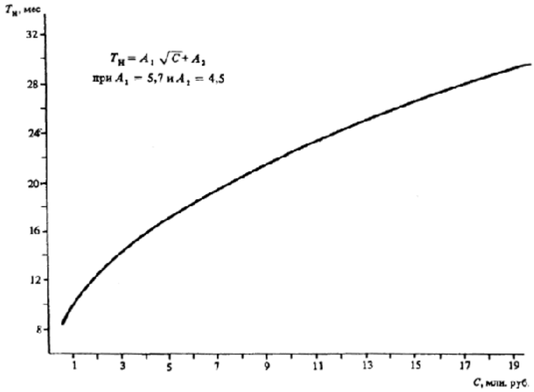
Черт. 26. Определение T_n различных объектов
