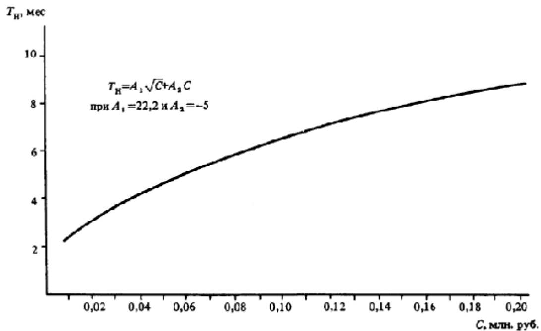
Черт. 47. Определение T_n прочих объектов
