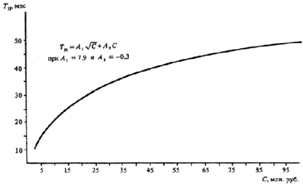
Черт. 37. Определение T_n различных объектов
