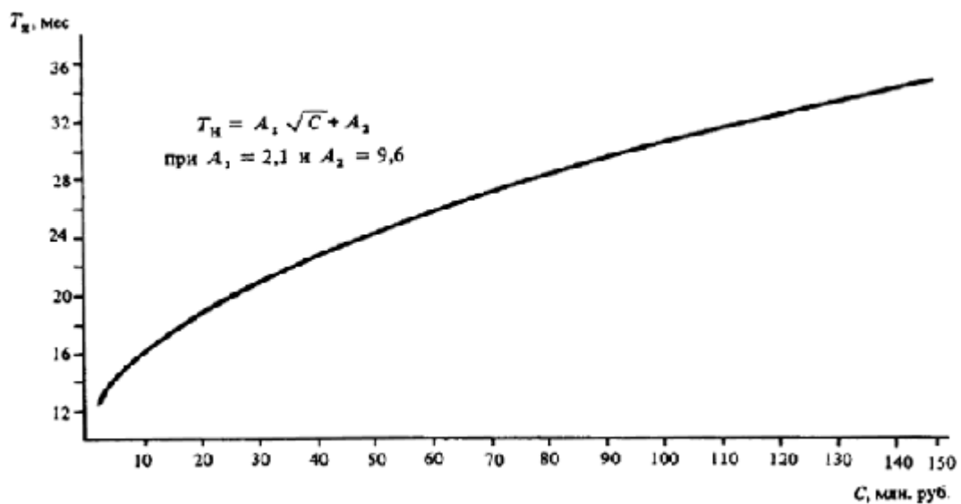
Черт. 8. Определение T_n горнообогатительных комбинатов и агломерационных фабрик
