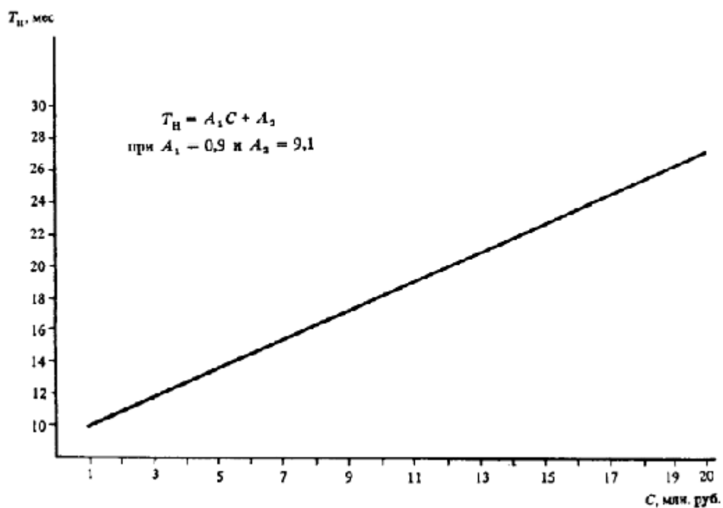
Черт. 2. Определение T_H ТЭЦ
