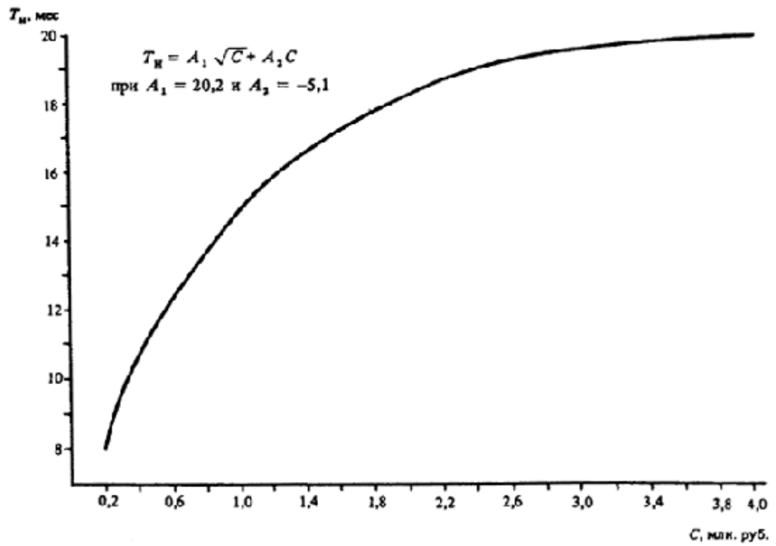
Черт. 60. Определение T_n общетоварных складов и предприятий холодильной промышленности
