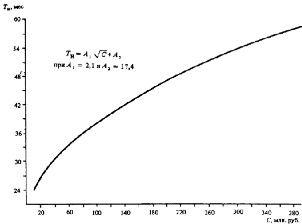
Черт. 24. Определение T_n различных объектов
