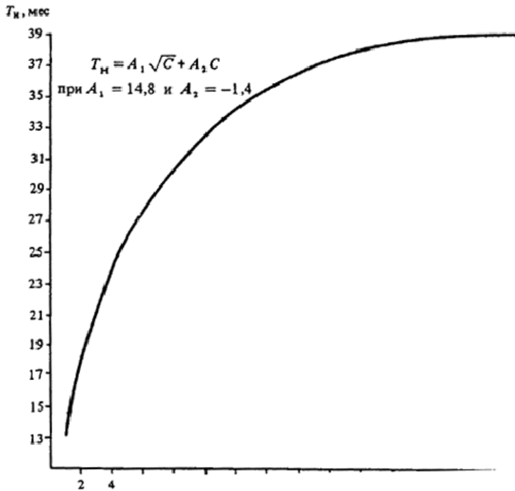
Черт. 33. Определение T_n различных объектов
