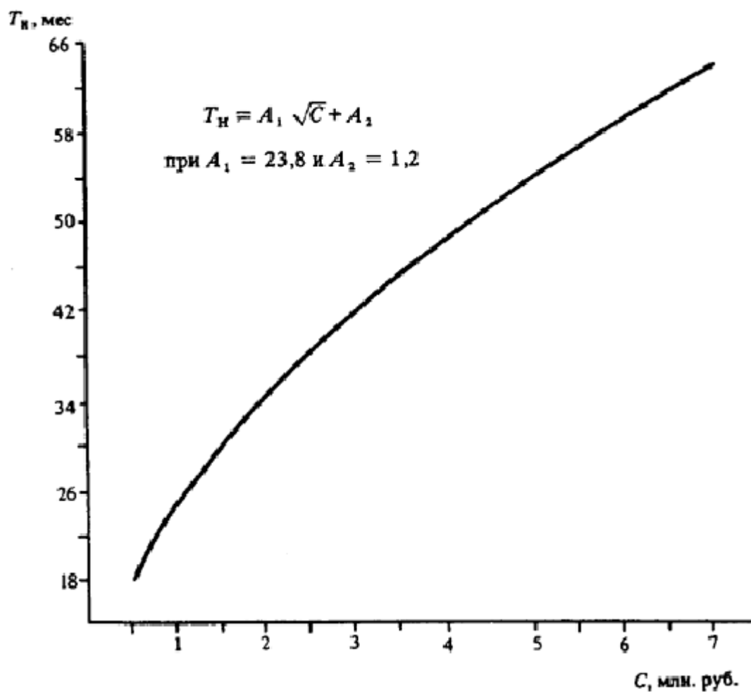
Черт. 57. Определение T_n различных объектов
