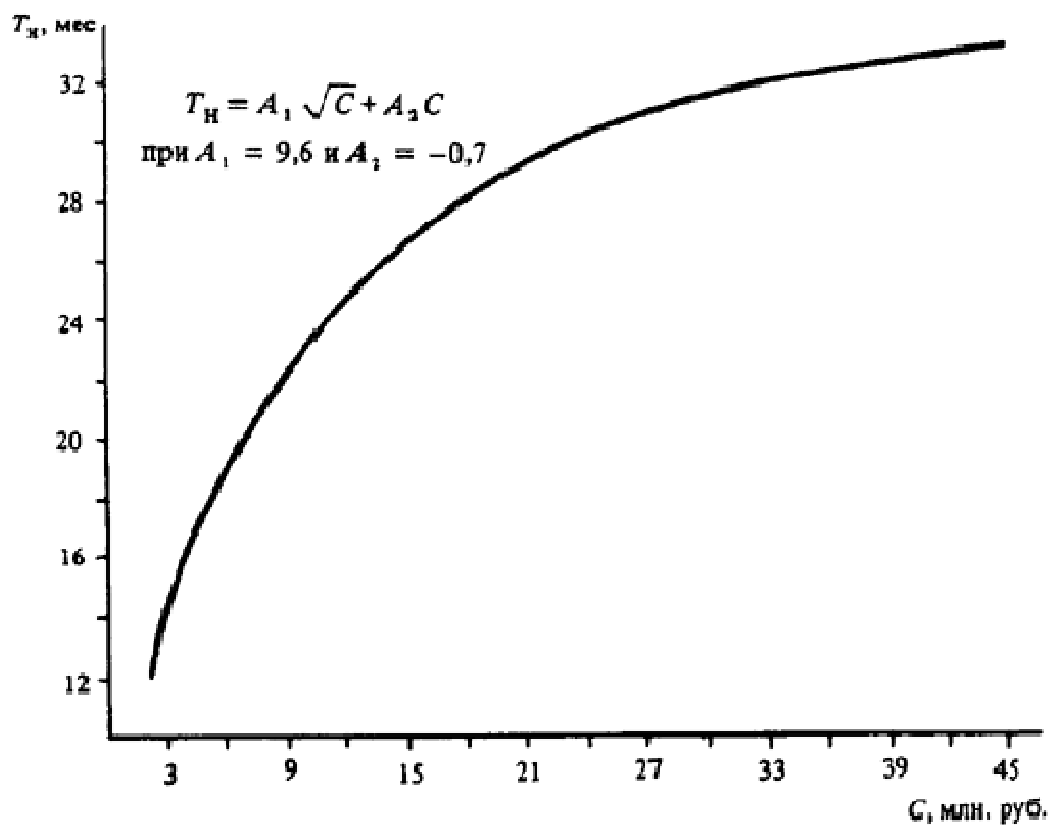
Черт. 14. Определение T_n различных объектов
