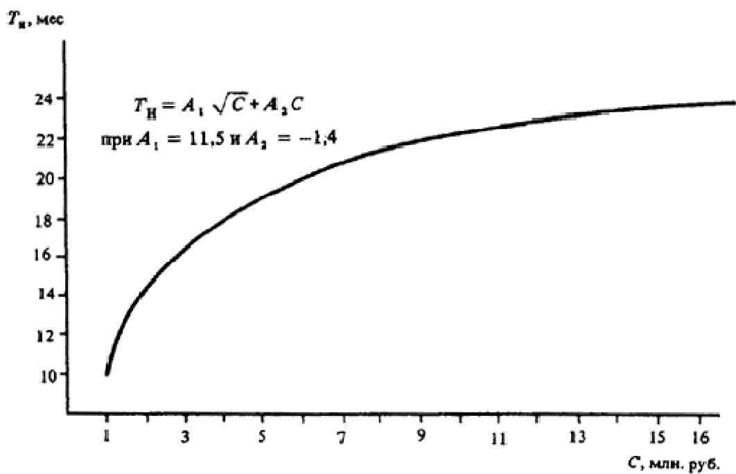
Черт. 22. Определение T_H отдельных цехов, корпусов и зданий
