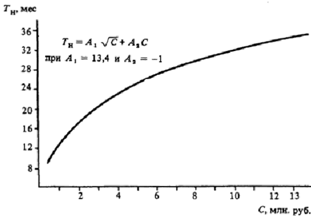
Черт. 50. Определение T_n различных объектов
