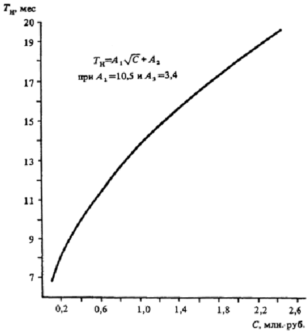
Черт. 43. Определение T_n овцеводческих ферм
