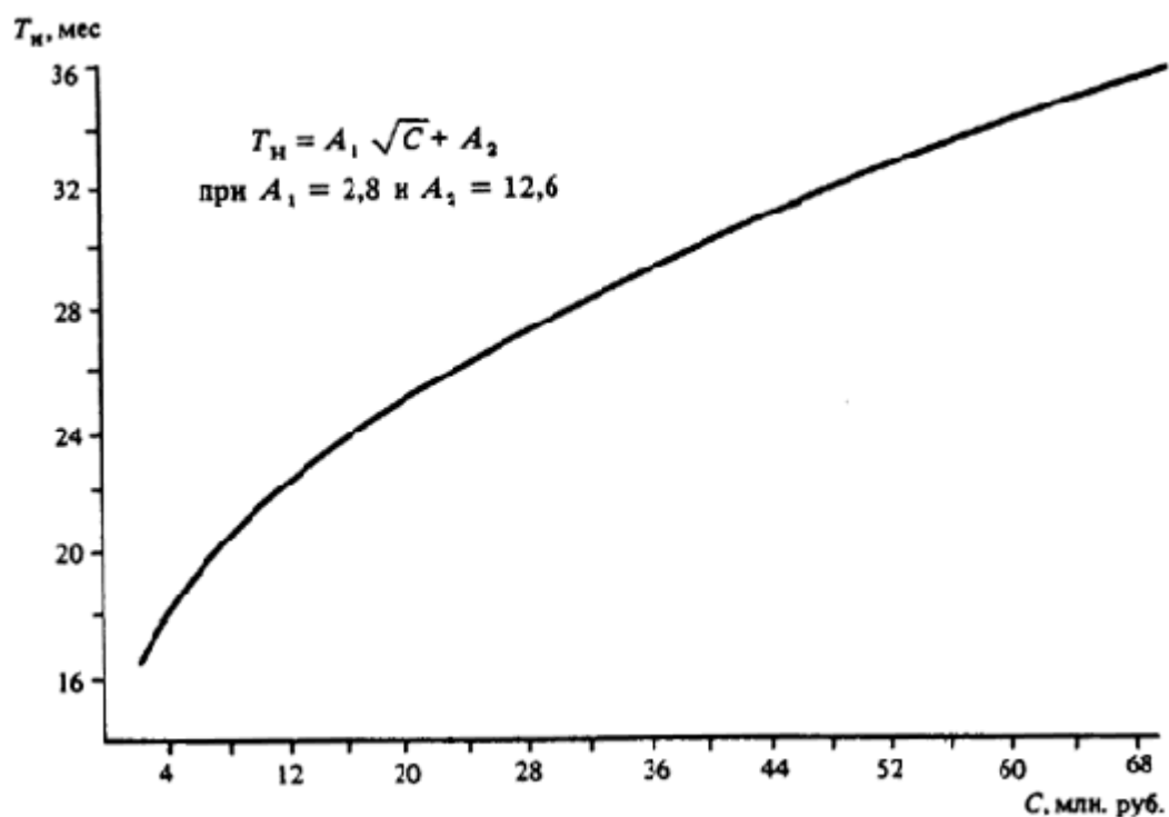
Черт. 12. Определение T_n различных объектов
