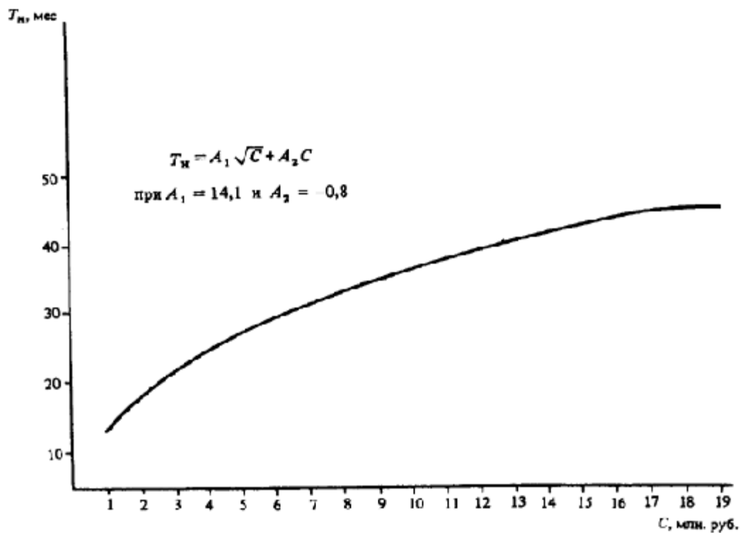
Черт. 34. Определение T_n различных объектов
