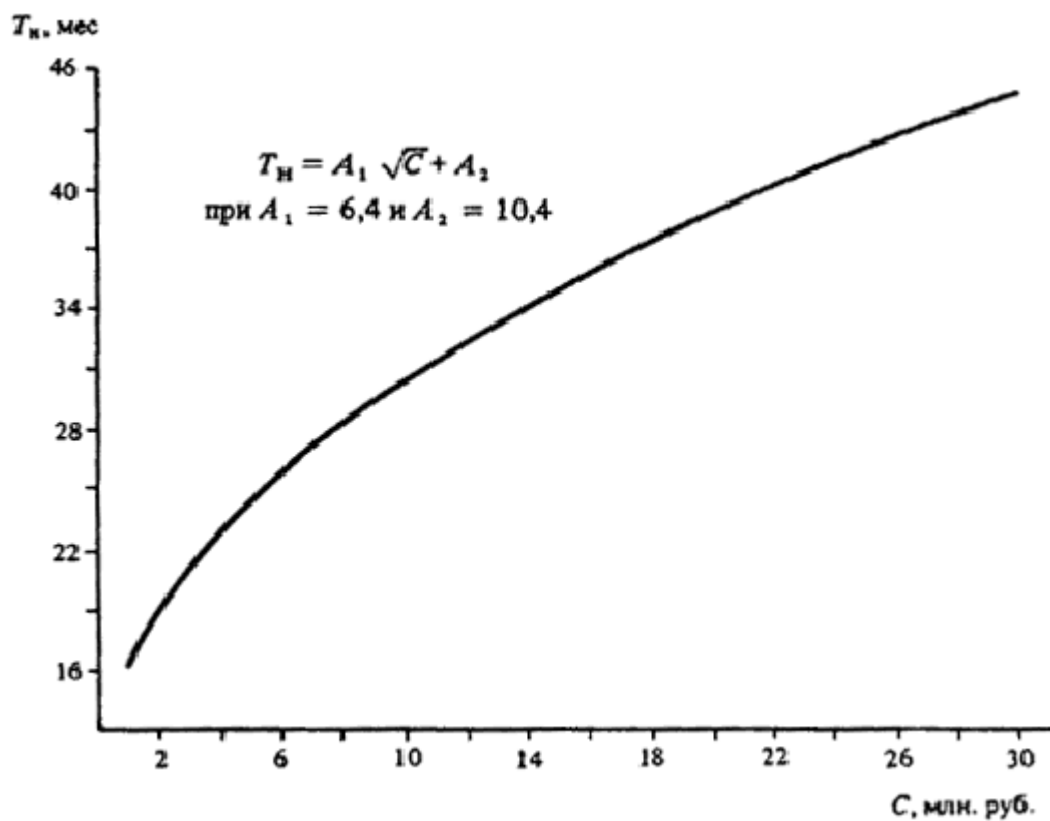
Черт. 31. Определение T_n различных объектов
