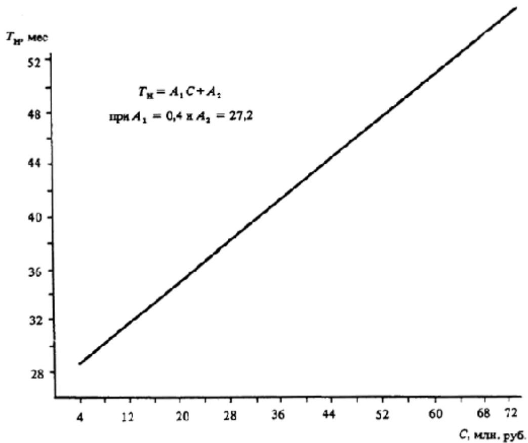
Черт. 19. Определение T_n различных объектов
