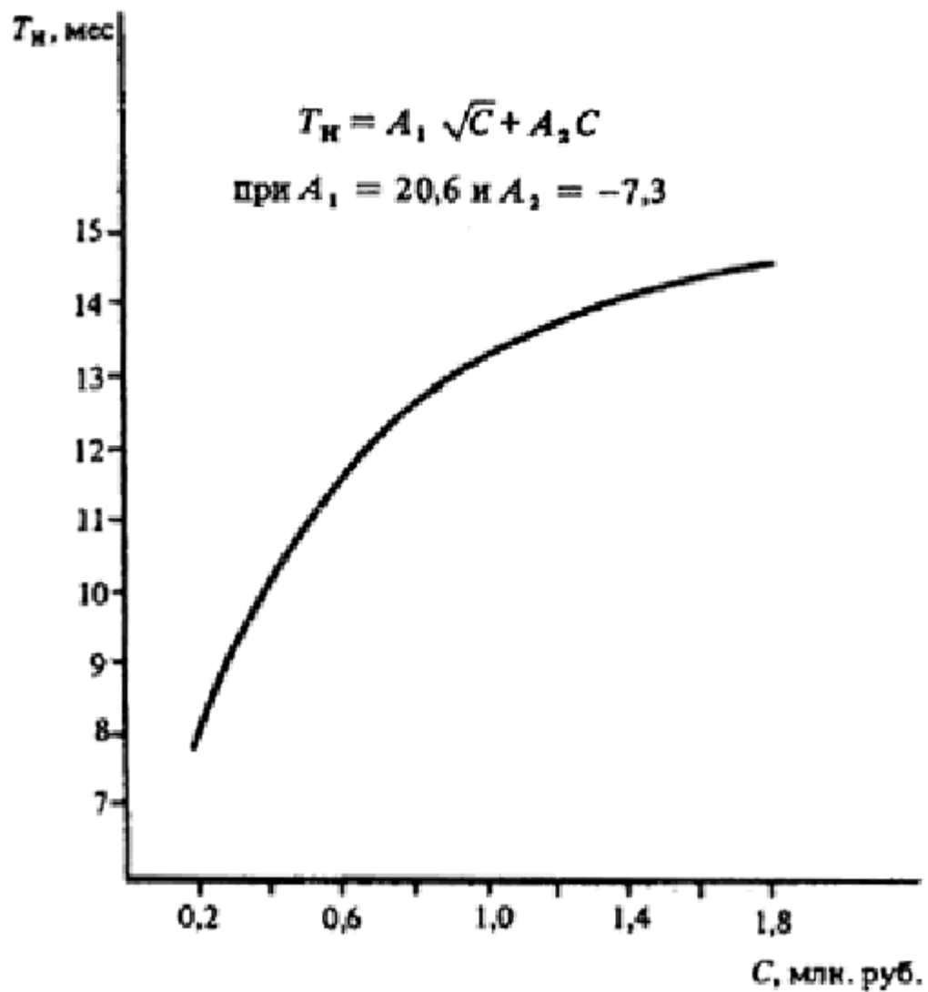
Черт. 54. Определение T_n объектов морского транспорта
