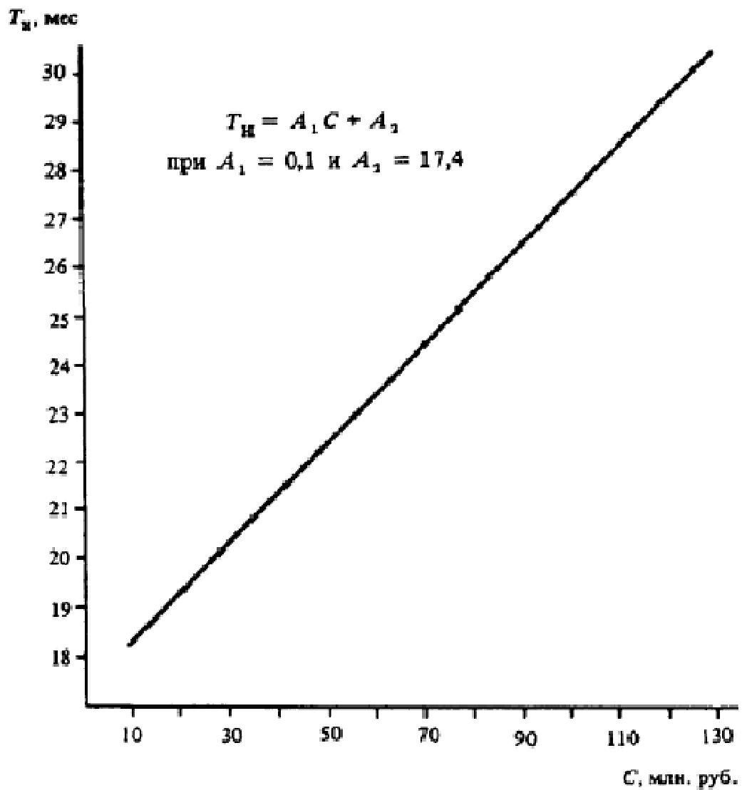
Черт. 10. Определение T_H объектов проката готовой продукции
