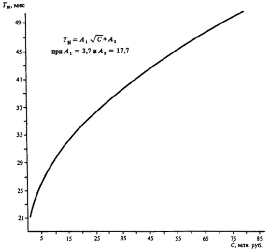
Черт. 15. Определение T_H различных объектов
