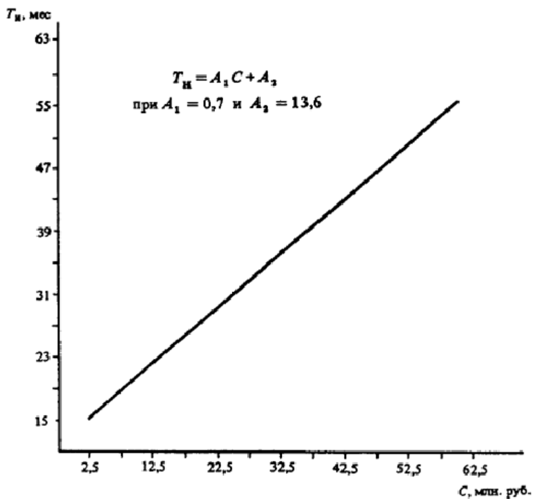
Черт. 39. Определение T_n различных объектов
