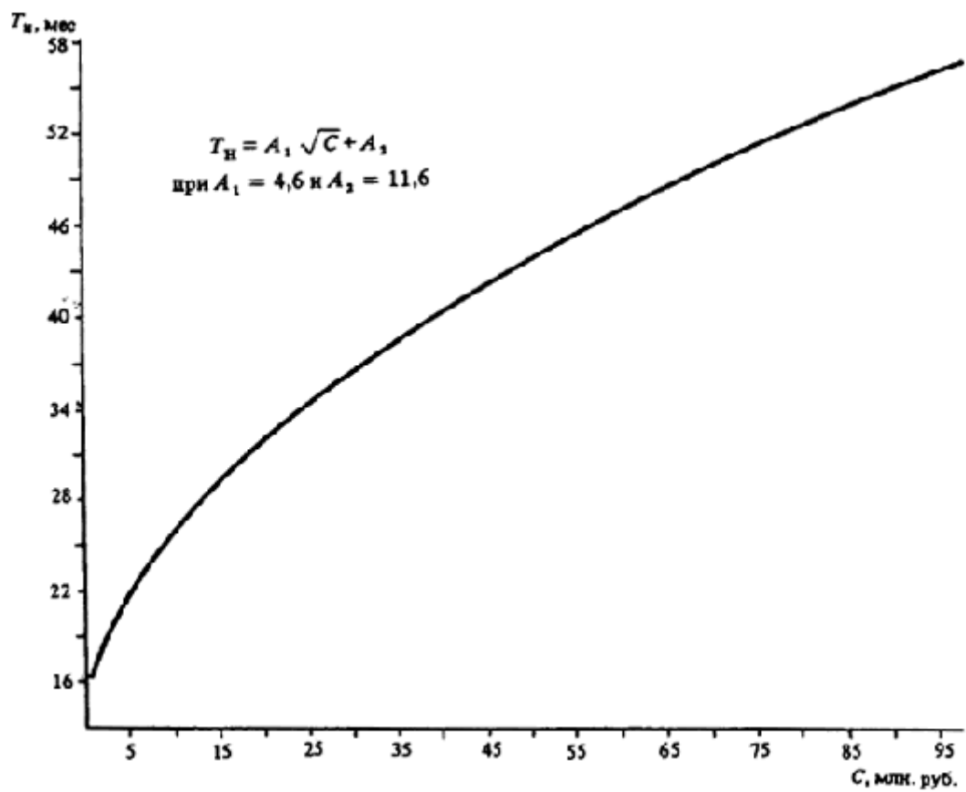
Черт. 28. Определение T_n различных объектов
