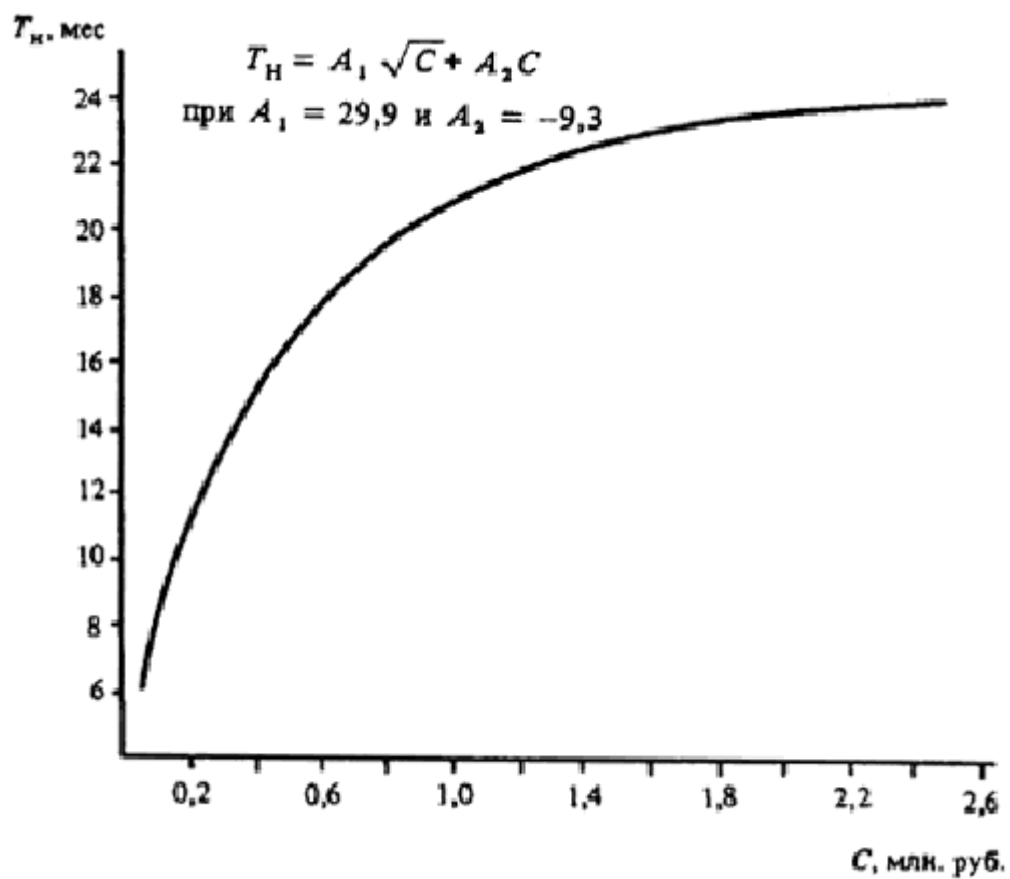
Черт. 58. Определение T_n объектов общественного питания и рынков
