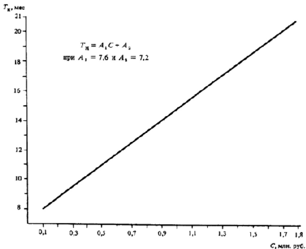
Черт. 6. Определение T_n баз производственного обслуживания
