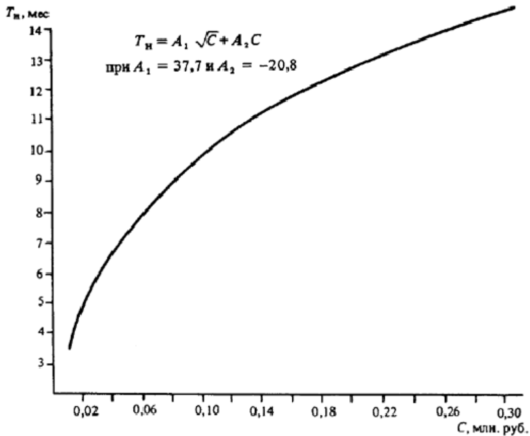
Черт. 52. Определение T_n различных объектов
