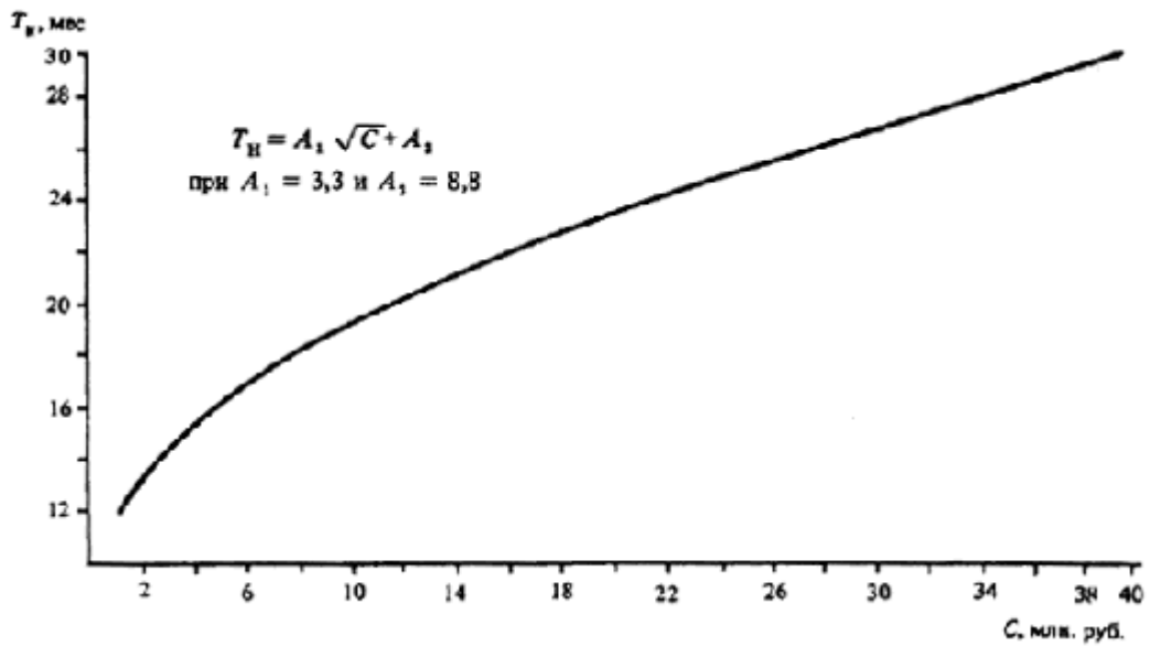
Черт. 7. Определение T_H различных объектов
