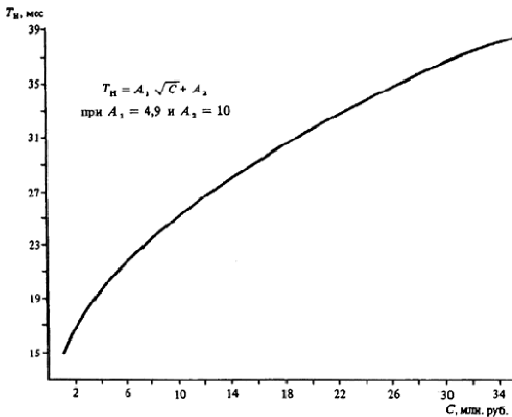
Черт. 32. Определение T_n различных объектов
