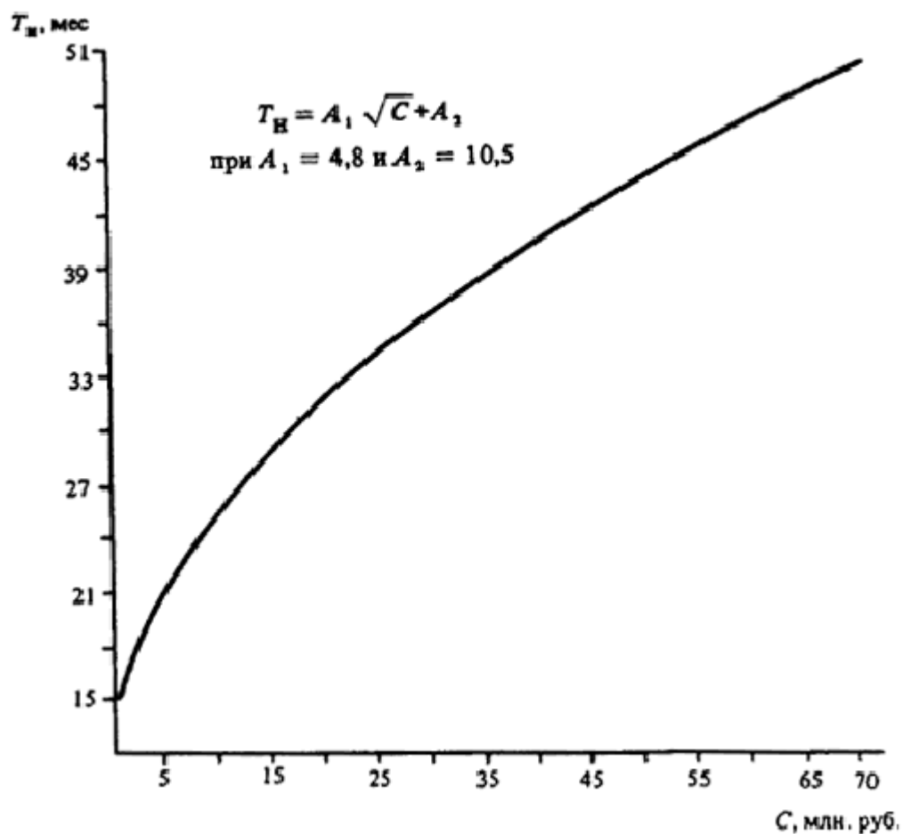
Черт. 13. Определение T_n различных объектов
