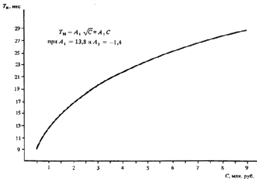
Черт. 61. Определение T_n различных объектов
