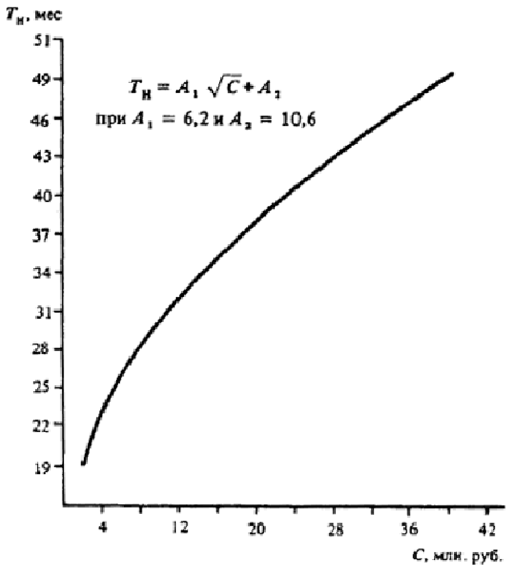
Черт. 21. Определение T_n различных объектов
