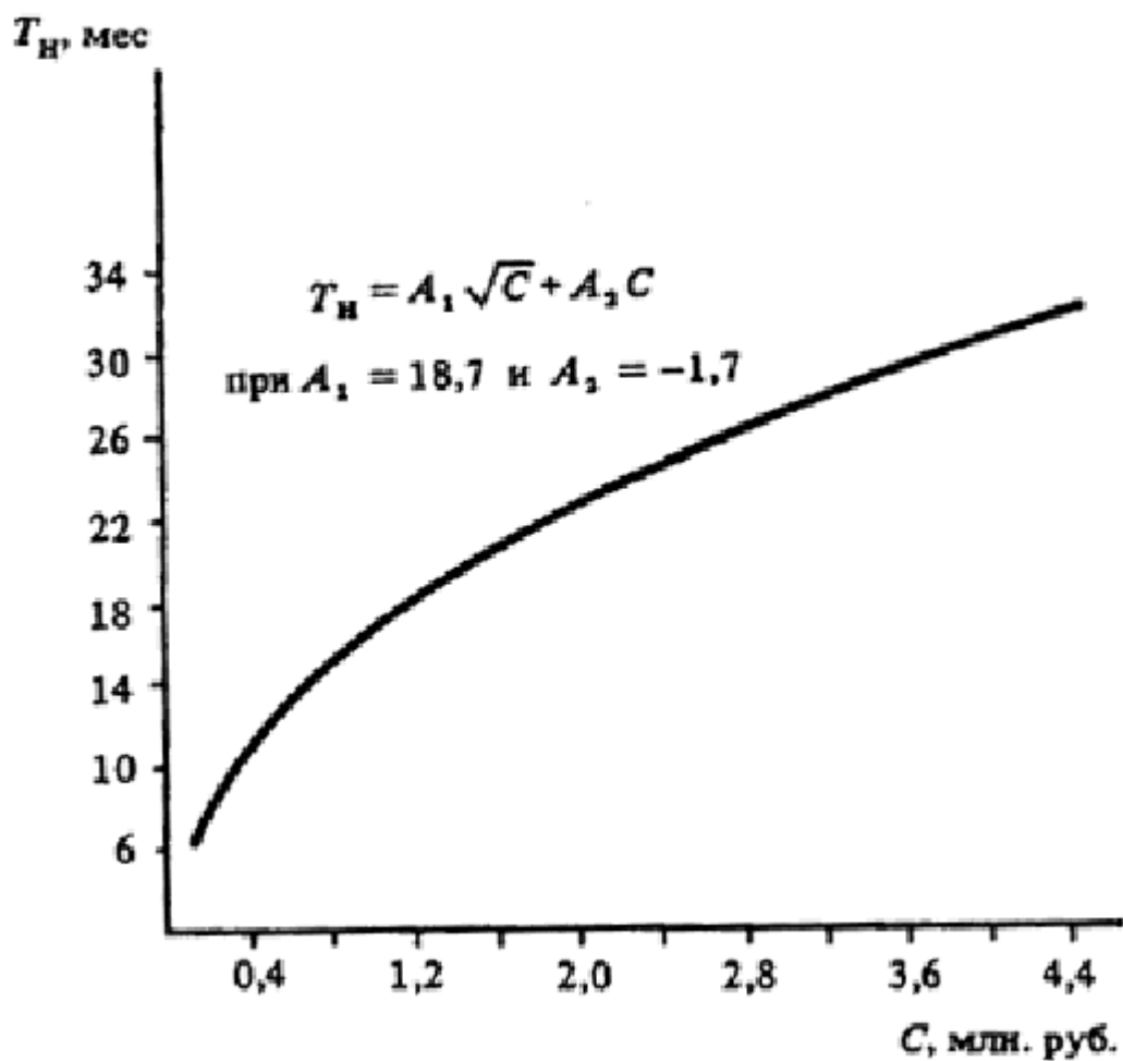
Черт. 35. Определение T_n разлитых объектов
