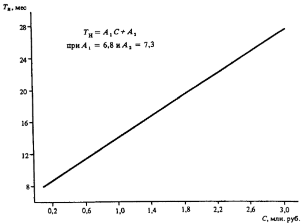
Черт. 48. Определение T_n предприятий по ремонту и обслуживанию сельхозтехники
