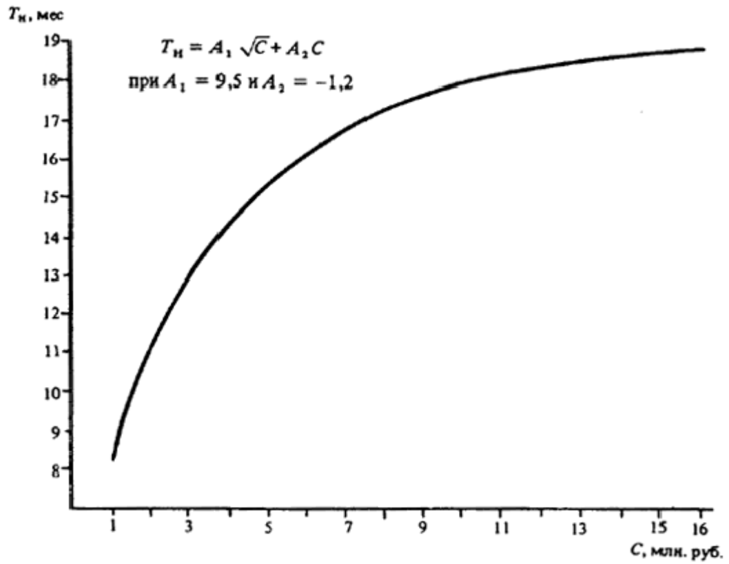
Черт. 56. Определение T_n различных объектов
