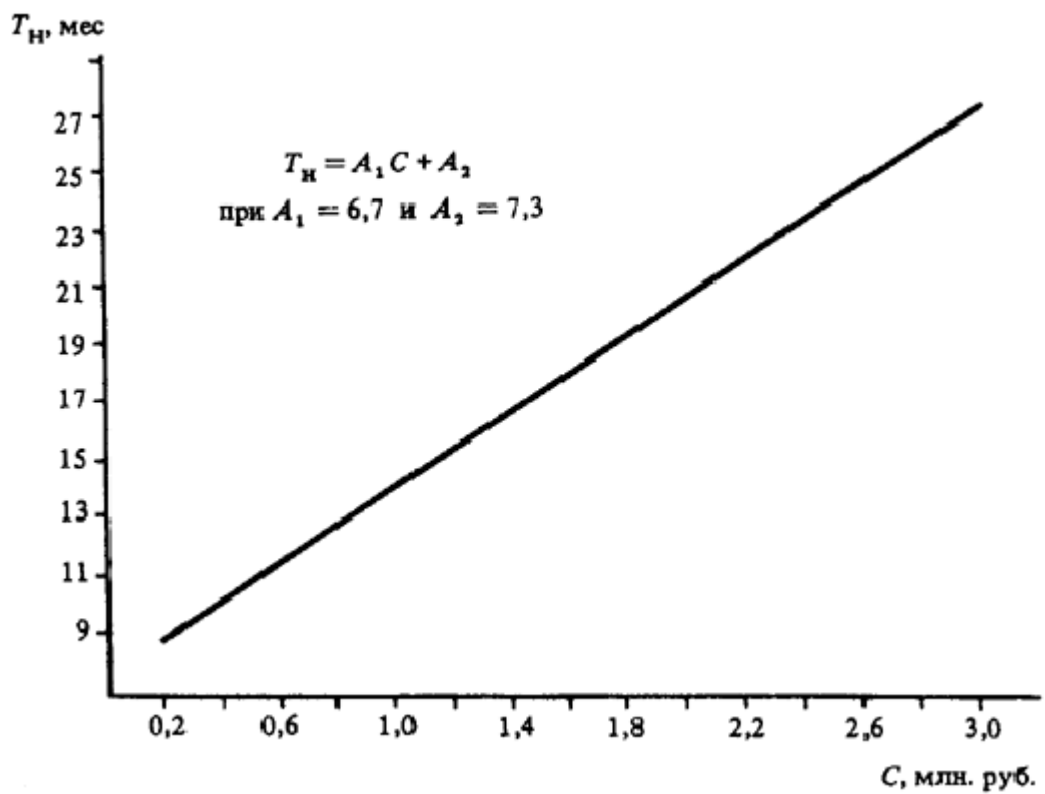
Черт. 40. Определение T_n различных объектов
