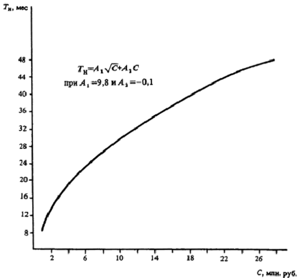
Черт. 45. Определение T_n птицеводческих ферм, птицефабрик
