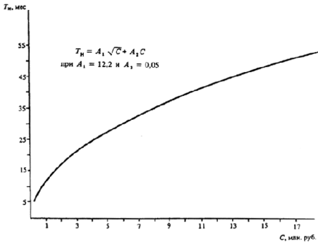
Черт. 38. Определение T_n различных объектов
