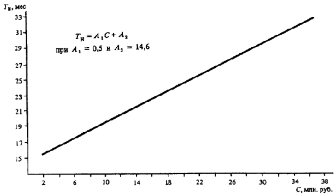
Черт. 20. Определение T_n различных объектов
