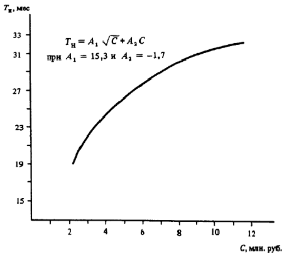
Черт. 4. Определение T_n электроподстанций
