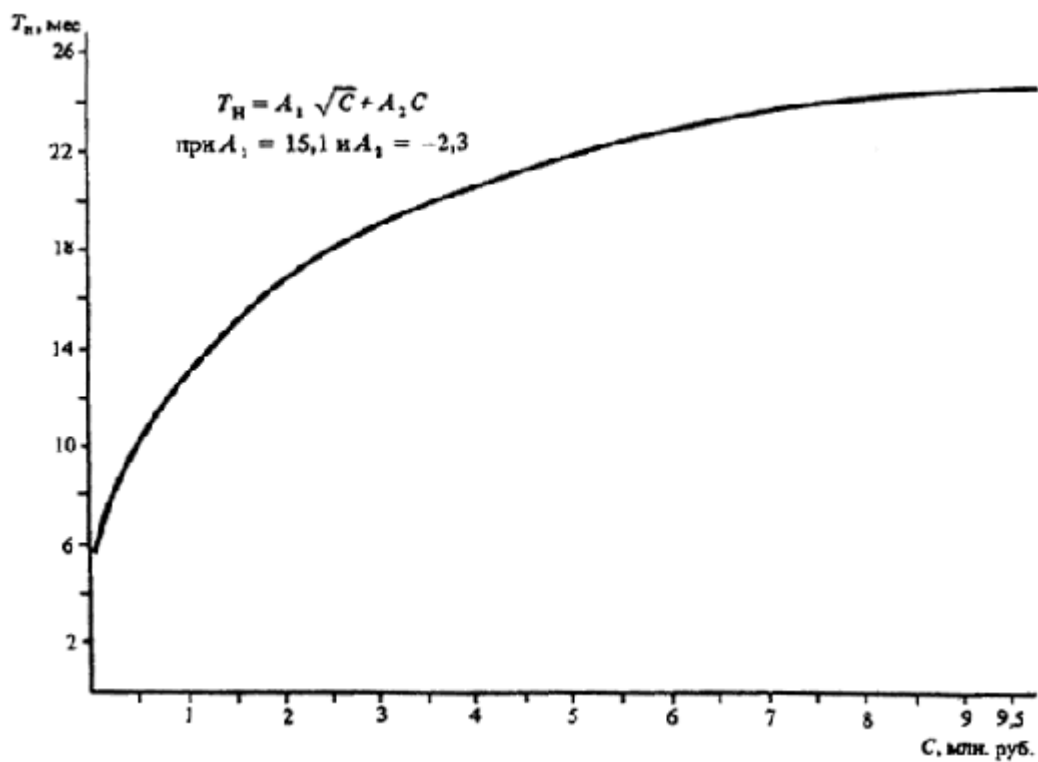
Черт. 30. Определение T_H различных объектов
