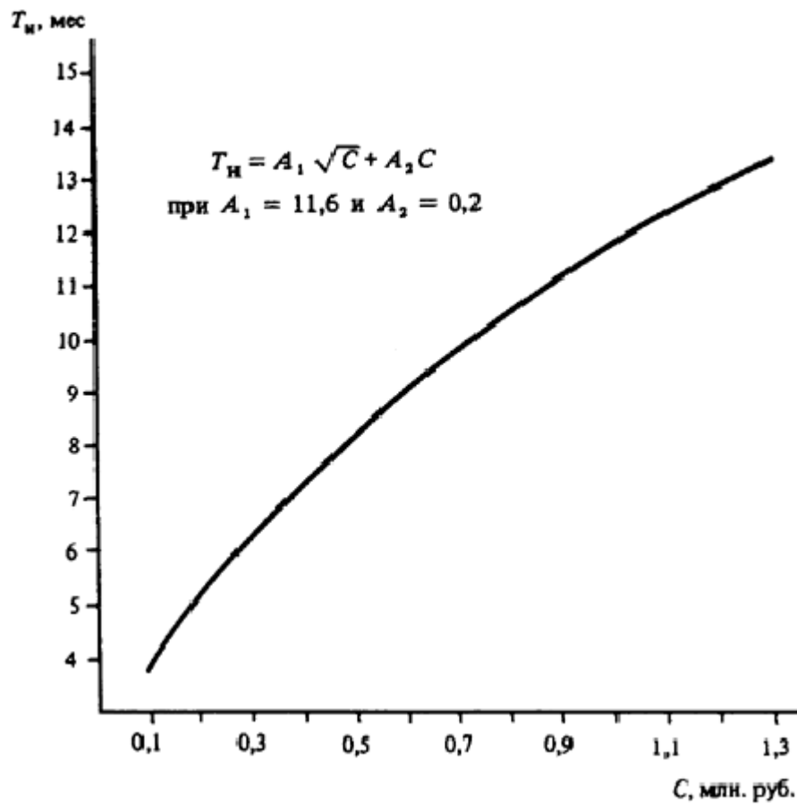
Черт. 3. Определение T_n электроподстанций
