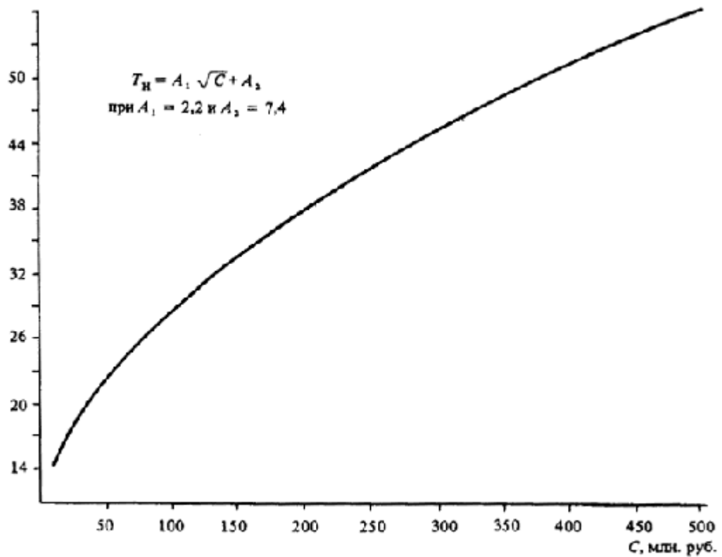
Черт. 29. Определение T_n различных объектов
