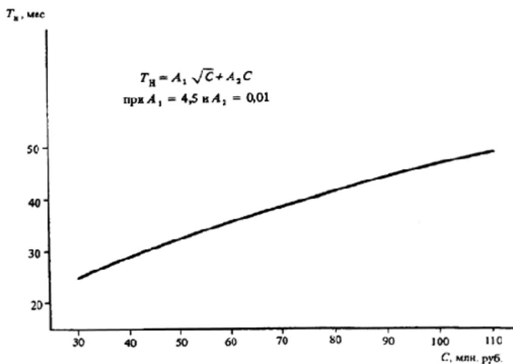
Черт. 1. Определение T_H ГРЭС
