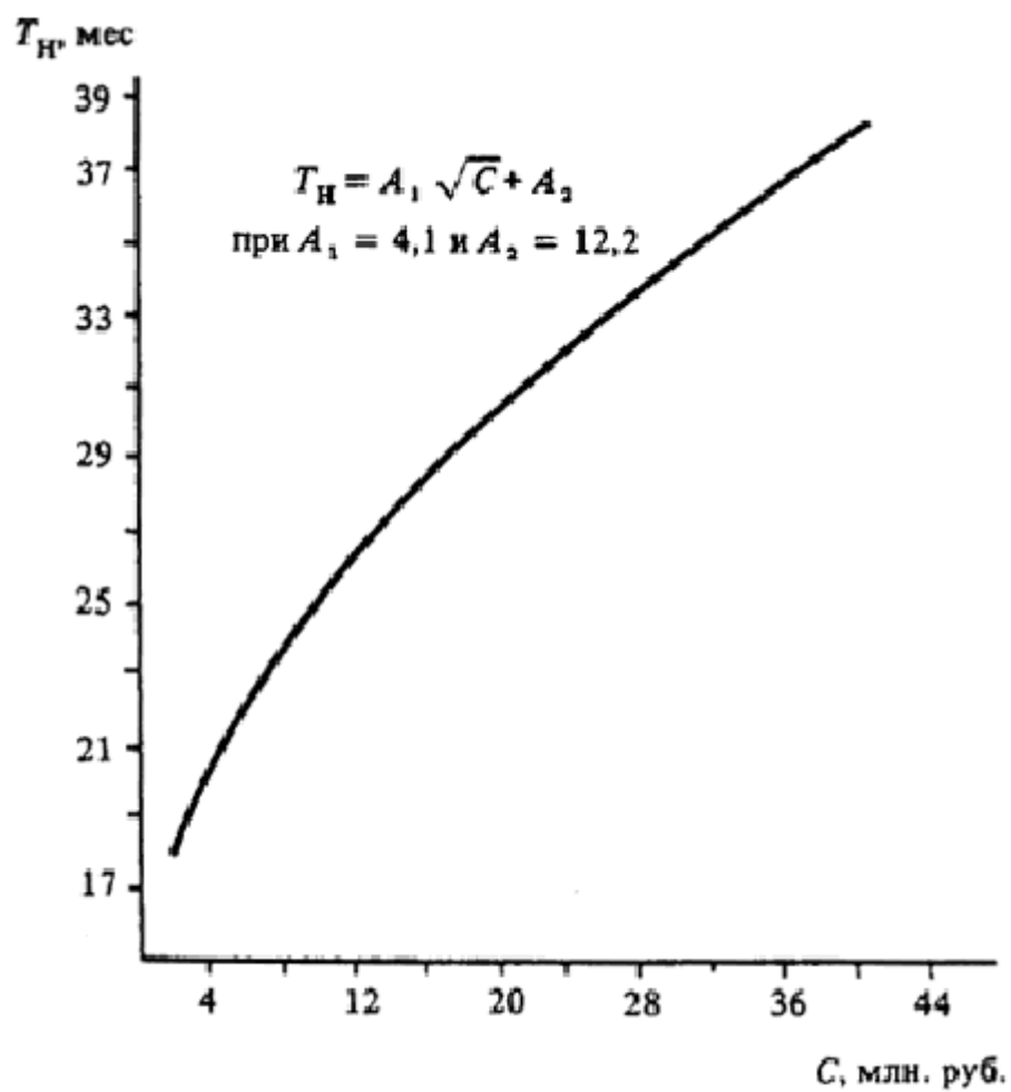
Черт. 17. Определение T_n различных объектов
