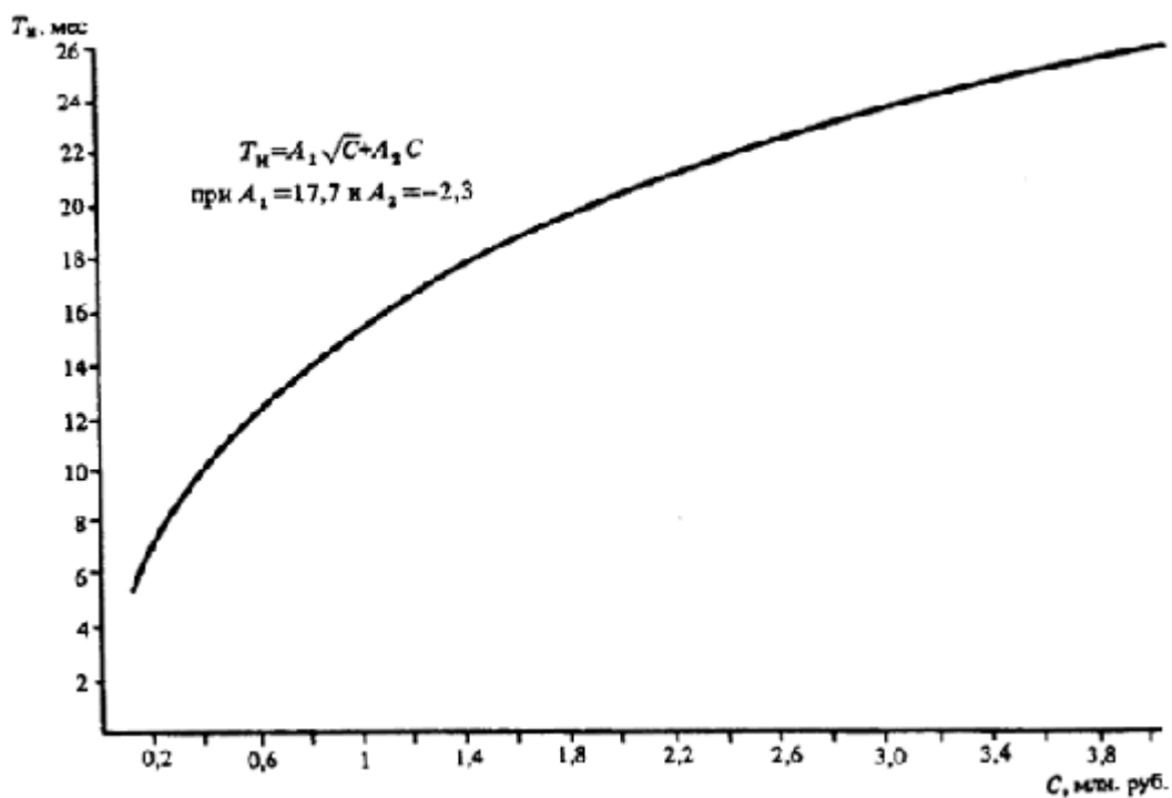
Черт. 44. Определение T_n объектов свиноводства
