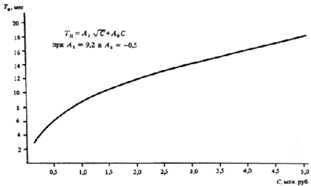
Черт. 5. Определение T_H установок подготовки, газокompрессорных при C = 0,1 - 6,0 млн. руб.
