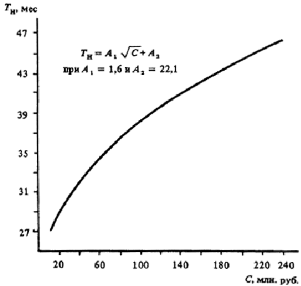
Черт. 23. Определение T_n различных объектов
