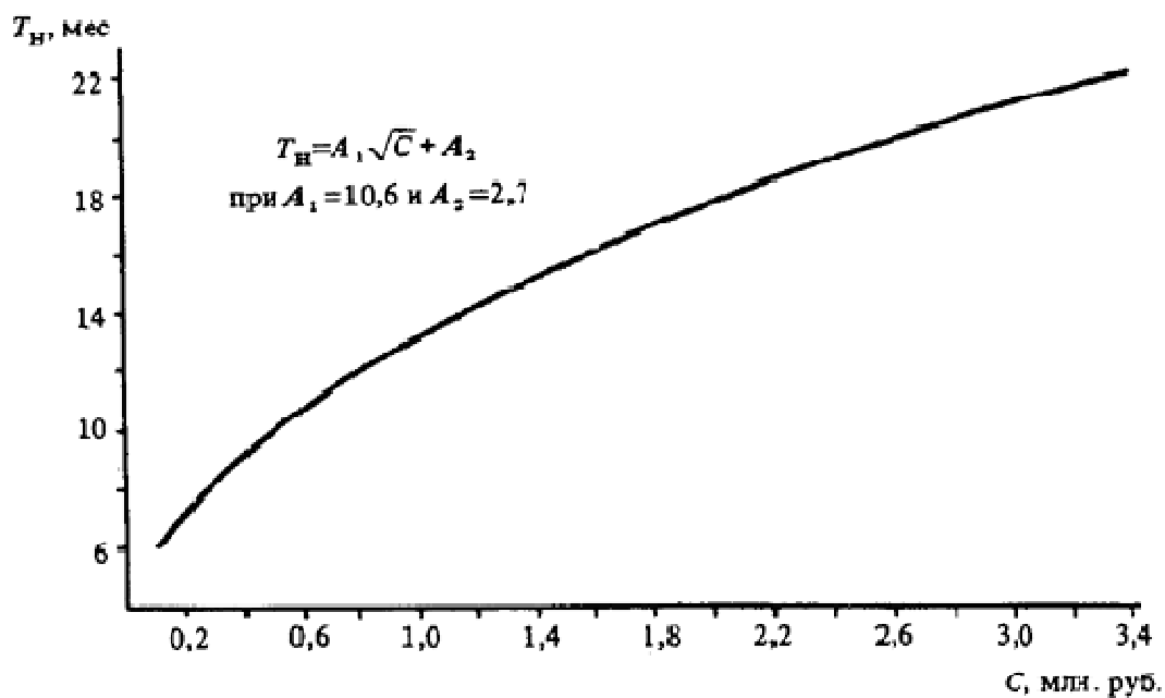
Черт. 42. Определение T_n объектов животноводства
