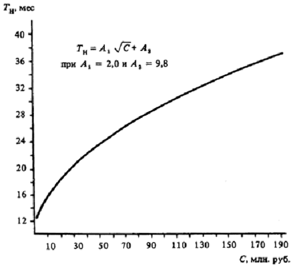
Черт. 11. Определение T_n объектов по отрасли в целом
