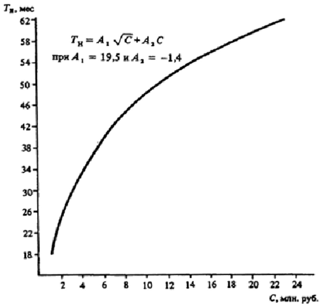
Черт. 27. Определение T_H лесозаготовительных предприятий
