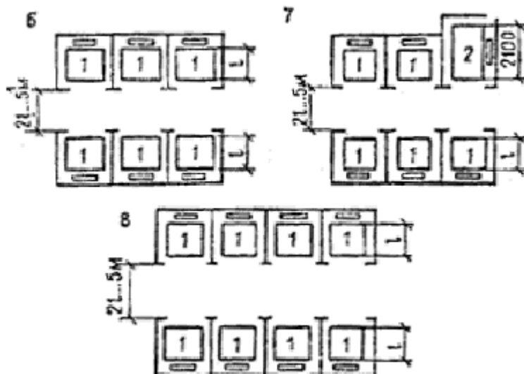
Рис. 8. Рекомендуемые сочетания и расположение пассажирских лифтов, объединяемых типовой системой группового управления. Сочетания 2б, г; 3б, г; 4б, г; 6б только для лифтов со скоростями 1 и 1,6 м/с
