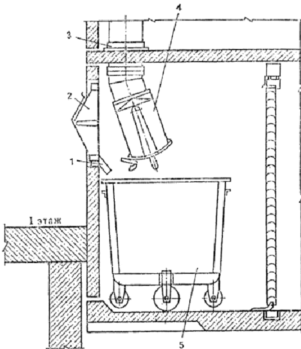
Рис. 14. Установка загрузочного клапана в стене мусоросборной камеры
