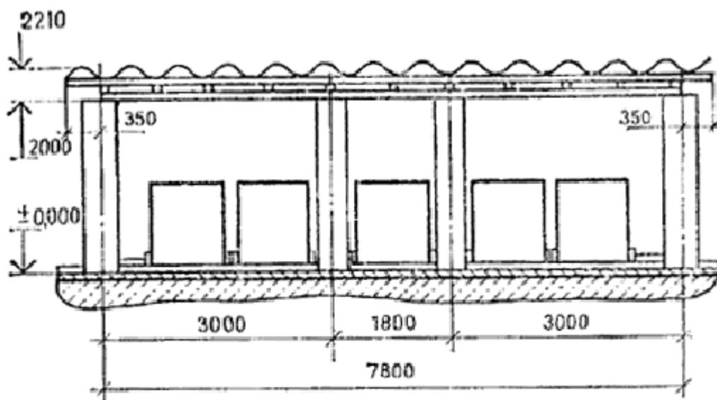
Рис. 19. Площадка крытая для двух контейнеров
