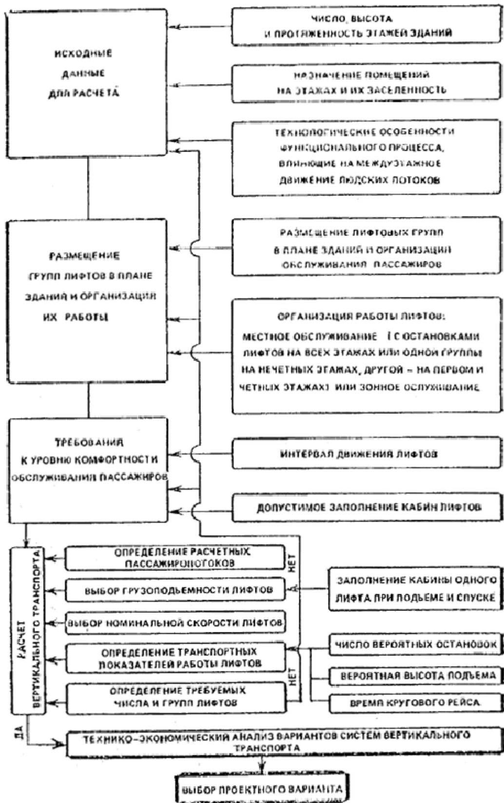
Блок-схема расчета вертикального транспорта
