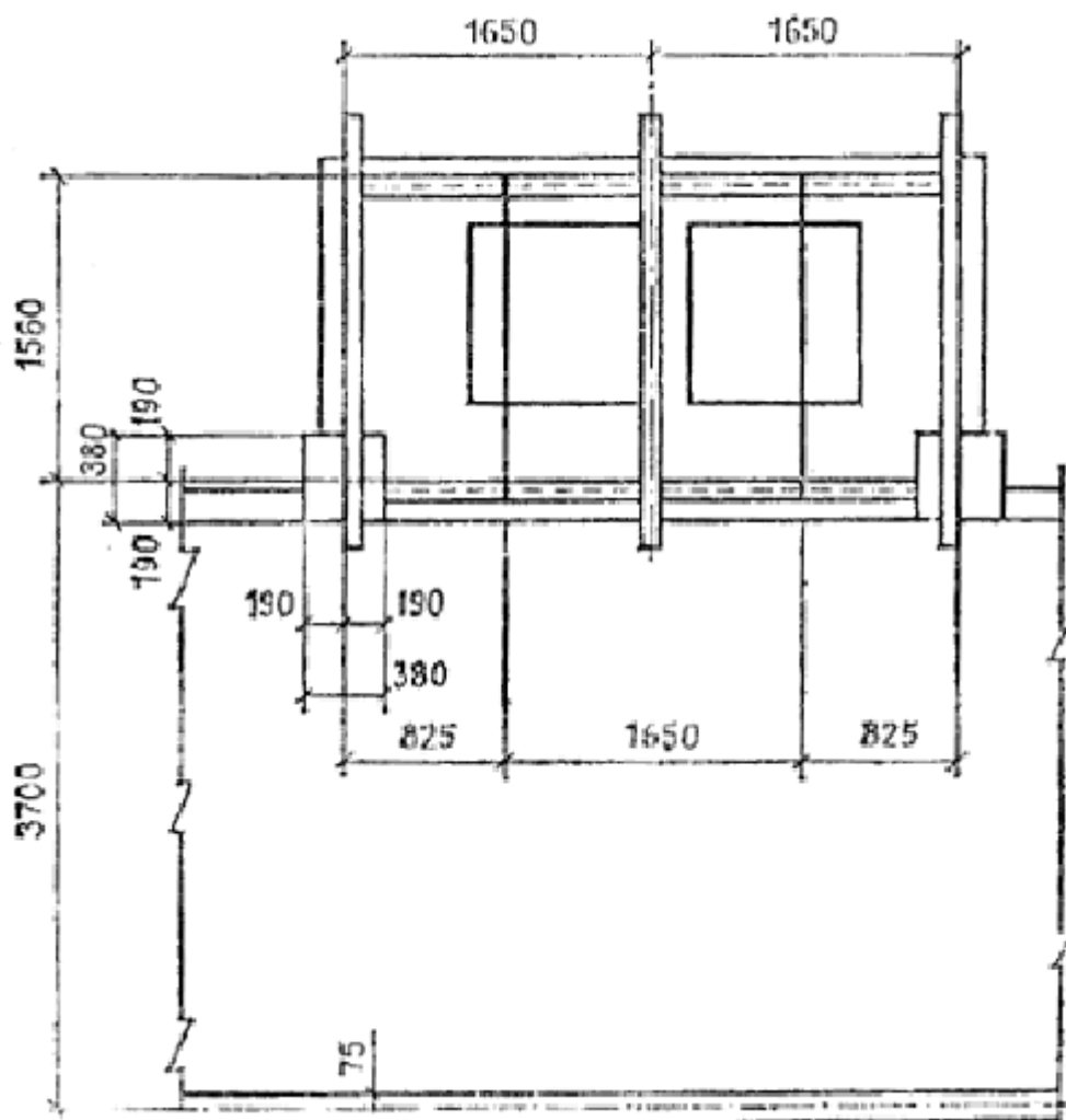
Рис. 19. Площадка крытая для двух контейнеров
