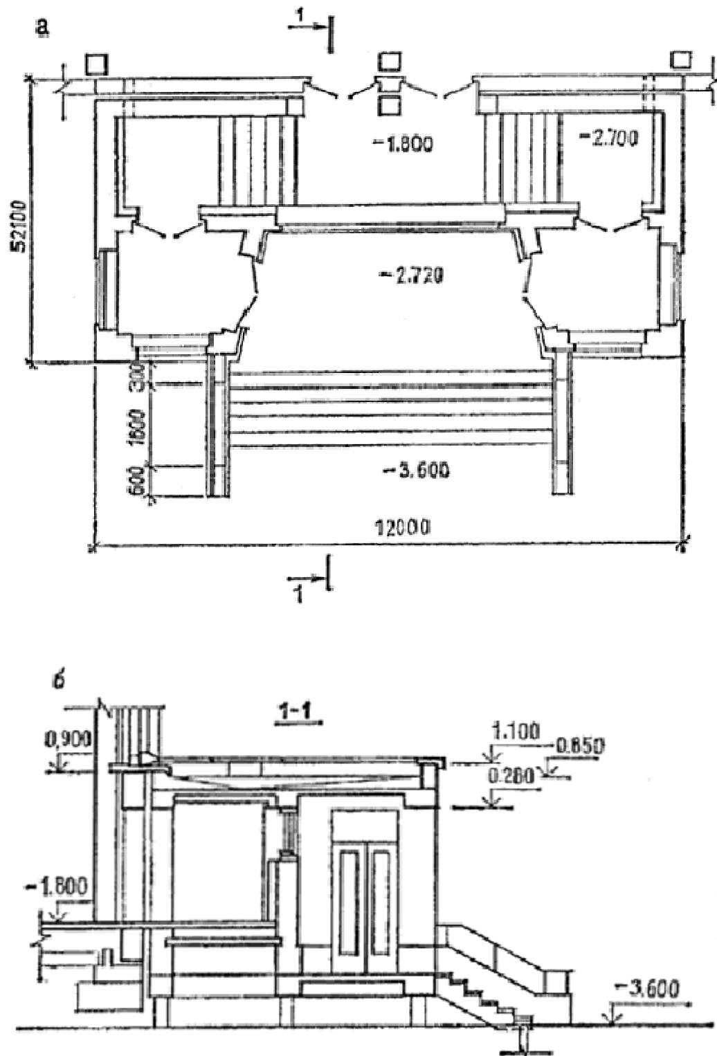
Рис. 4. Решение входа в здание (на примере общественного центра) с устройством двойного тамбура: а — план; б — разрез
