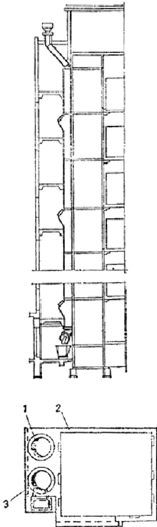
Рис. 15. Схема ствола мусоропровода, совмещенного с лифтовой шахтой
