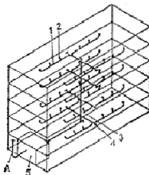
Рис. 12. Схема вакуумной централизованной пылеборки с вертикальным магистральным пылепроводом
