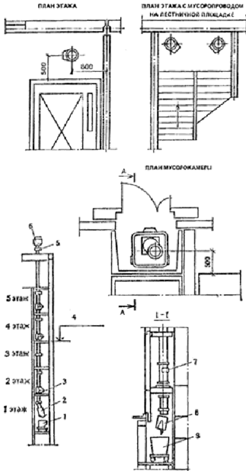
Рис. 13. Примерные схемы мусоропроводов
