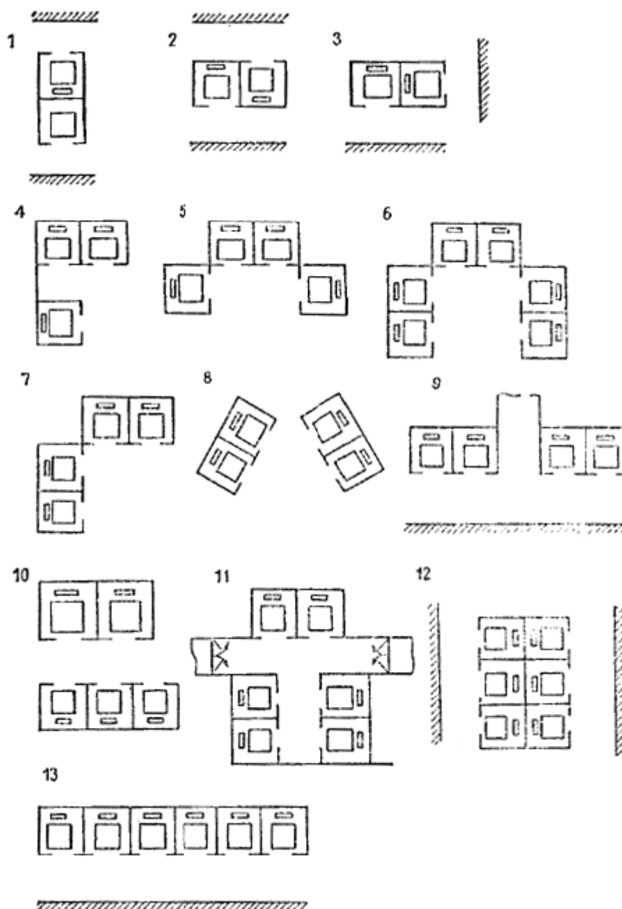
Рис. 9. Примеры схем нерекондуемого расположения лифтов
