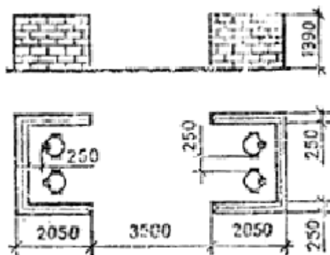
Рис. 18. Схема площадки под мусоросборники вместимостью 0,1 м 3
