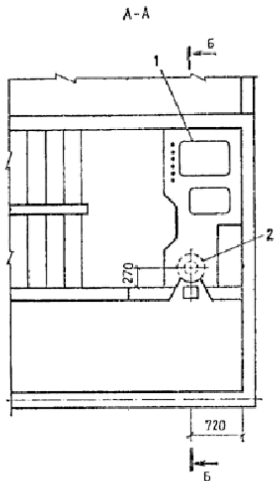
Рис. 16. Схема ствола мусоропровода, совмещенного с вентиляционным блоком
