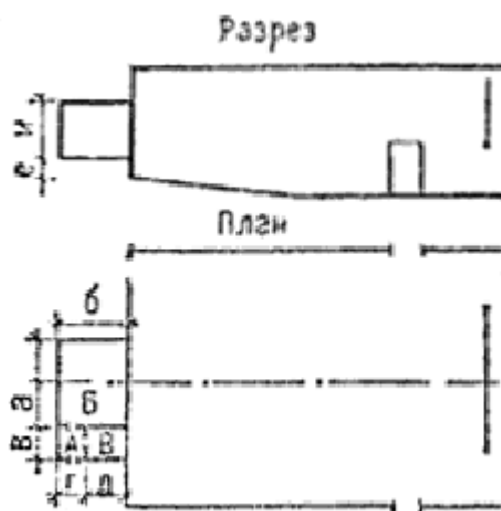
Рис. 6. Схема планировки кинопроекционного комплекса конференц-зала
