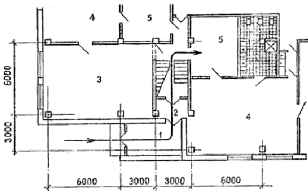
Рис. 5. Решение входа в здание (на примере детских яслей-сада) с устройством двойного тамбура
