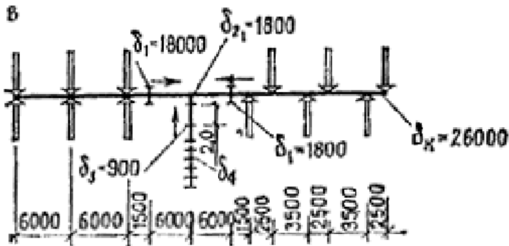
Схема плана типового этажа технического вуза
