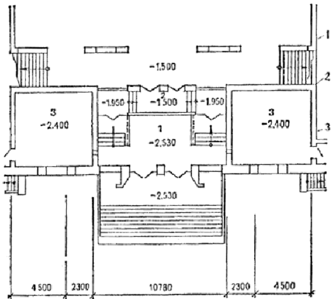
Рис. 3. Фрагмент (вход в здание)
