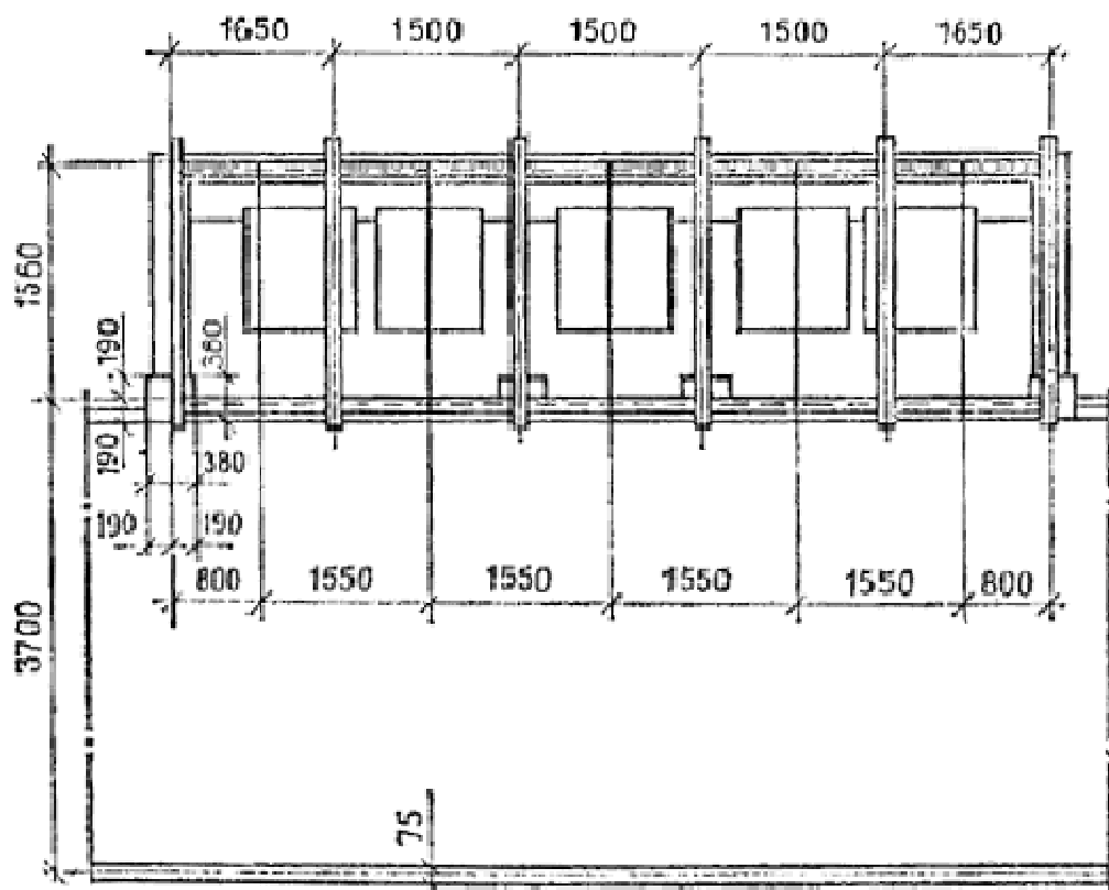
Рис. 20. Площадка крытая для пяти контейнеров
