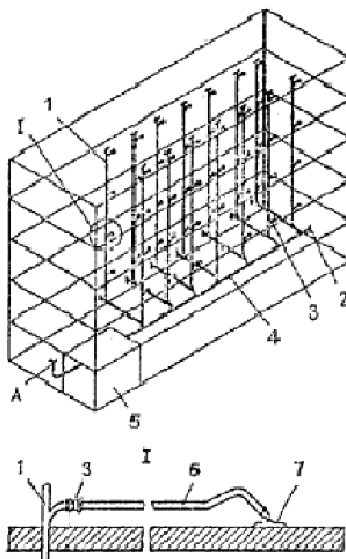
Рис. 11. Схема вакуумной централизованной пылеборки с горизонтальным магистральным трубопроводом
