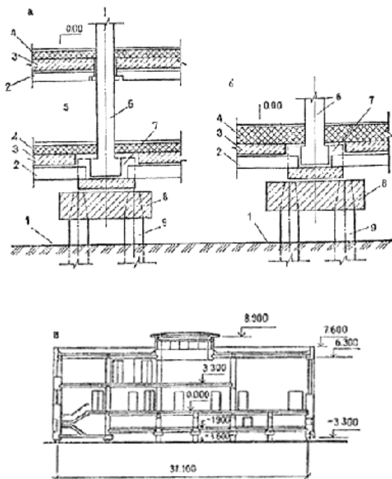
Рис. 1. Цокольно-фундаментная часть здания каркасной конструкции (1 принцип строительства)
