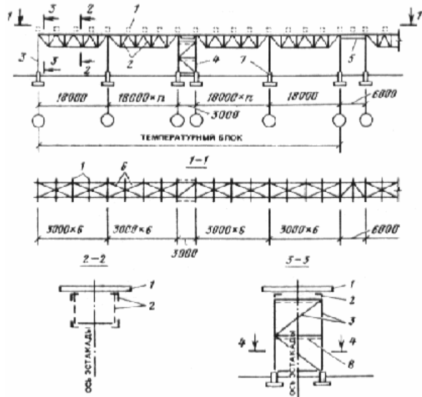
Рис. 7. Конструктивная схема одноярусной стальной эстакады
