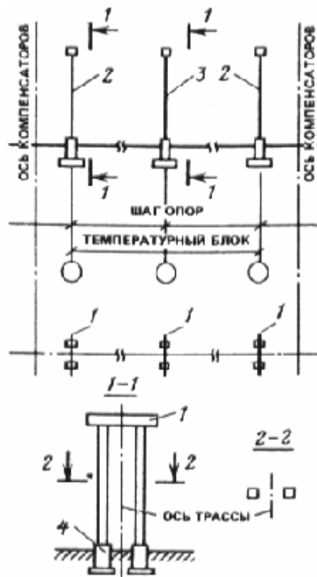
Рис. 3. Конструктивная схема отдельно стоящих железобетонных опор
