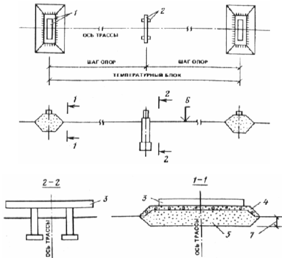
Рис. 2. Конструктивная схема шпальных отдельно стоящих опор
