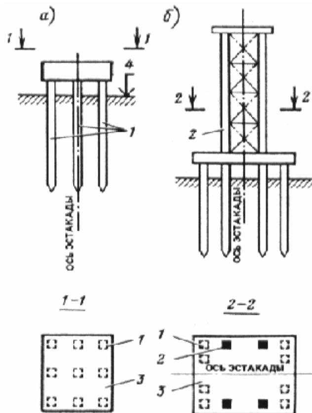
Рис. 13. Опоры с применением свайного ростверка
