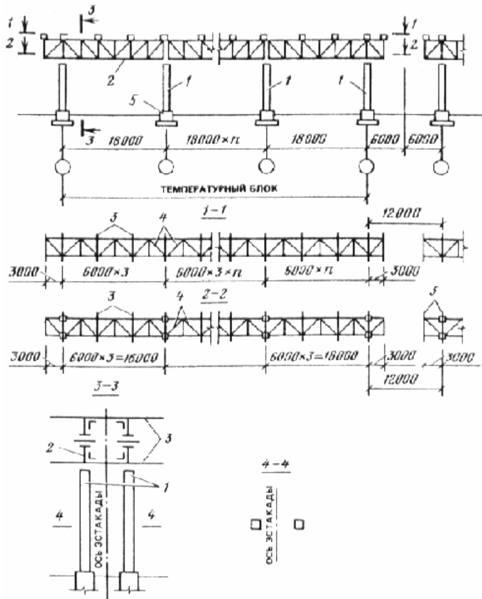
Рис. 6. Конструктивная схема двухъярусной эстакады
