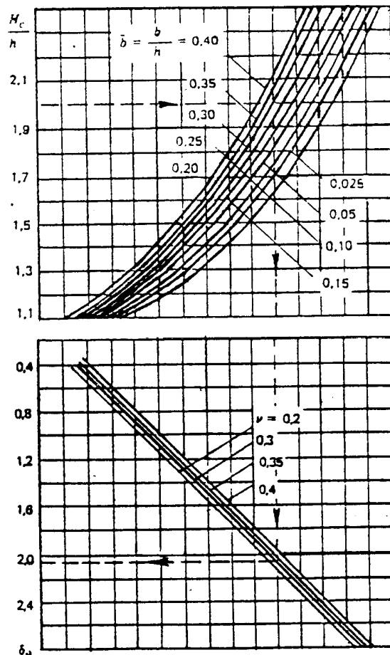
Номограмма для определения значений \delta_0
