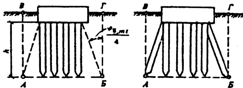
Определение границ условного фундамента при расчете осадок свайных фундаментов
