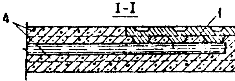
Черт.17. Приварка к концам стержней анкерующих пластин или закладных деталей 1 — пластина (рифленая в местах контактной сварки) ; 2 — рабочие стержни ненапрягаемой арматуры; 3 - место точечной электросварки; 4 — сетки
