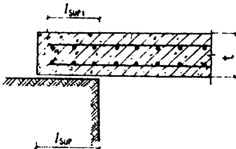
Черт. 16. Схема свободного опирания плоских нагибаемых элементов
