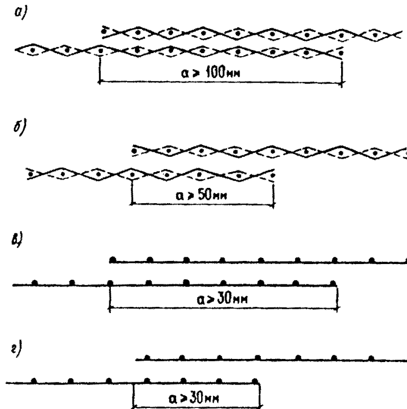
Черт. 18. Стыки сеток, выполняемые внахлестку
