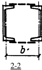
Черт. 4. Составной стержень на планках
