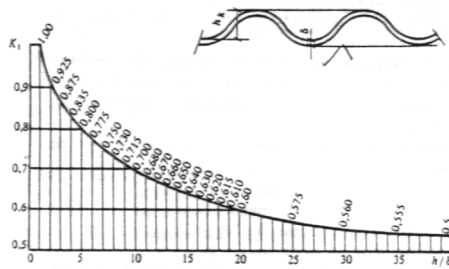
Черт.7. График для определения коэффициента K_I
