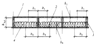
Черт.2. Поперечное сечение каркасной плиты
