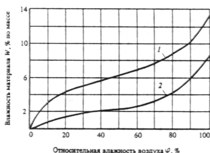
Черт.9. Зависимость влажности W листового 1 и экструзионного 2 асбестоцементов от относительной влажности воздуха \varphi .
