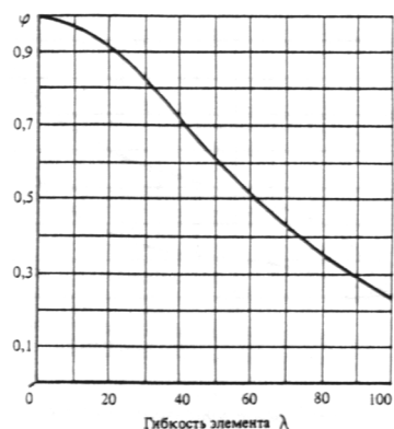
Черт.10. График определения коэффициента продольного изгиба \varphi .
