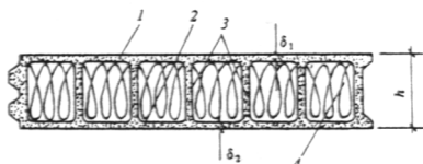
Черт.4. Поперечное сечение экструзионной панели
