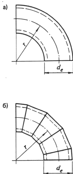
Черт. 4. Отводы а — бесшовный и штампосварной; б — сварной
