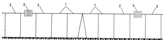
Схема прокладки трубопровода на опорах
