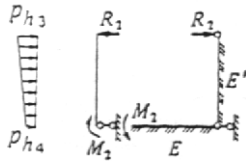
Черт. 4. Расчетная схема тоннеля с шарнирами в уровне плит перекрытия
