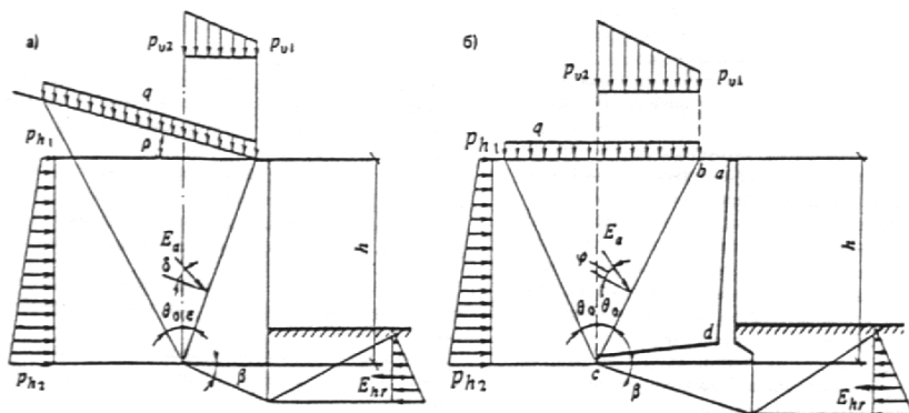
Черт. 1. Расчетные схемы подпорных стен a — массивных; б — углового профиля
