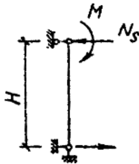
Рис. 12. Определение усилия в анкере от изгибающего момента в уровне перекрытия
