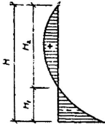
Рис. 6. Знакопеременная эпюра изгибающего момента для внецентренно сжатого элемента
