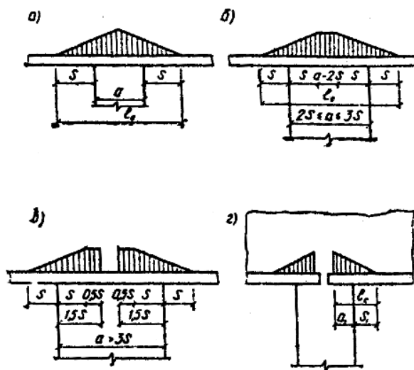
Рис. 15. Распределение давления в кладке над опорами висячих стен a - на средних опорах неразрезных балок при a \leq 2s ; б - то же, при 3s \geq a > 2s ; в - то же, при a > 3s ; г - на крайних опорах неразрезных балок и на опорах однопролетных рандбалок
