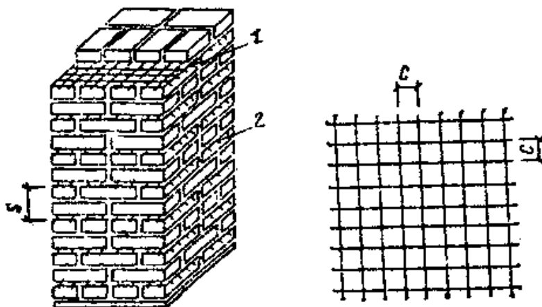
Рис. 10. Поперечное (сетчатое) армирование каменных конструкций 1 - арматурная сетка; 2 - выпуск арматурной сетки для контроля ее укладки
