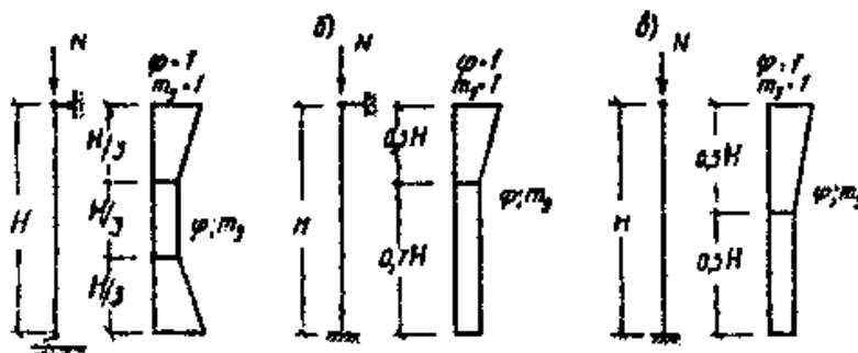
Рис. 4. Коэффициенты \varphi и m_g по высоте сжатых стен и столбов а - шарнирно опертых на неподвижные опоры; б - защемленных внизу и имеющих верхнюю упругую опору; в - свободно стоящих
