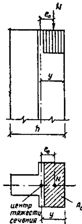
Рис. 5. Внецентренное сжатие
