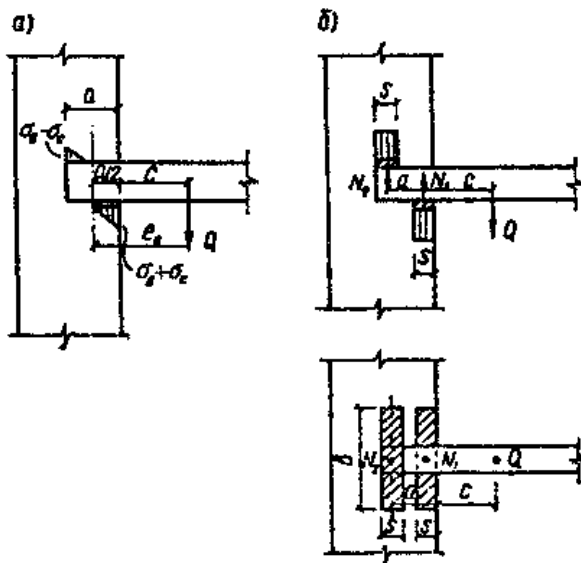
Рис. 14. Расчетные схемы заделки консольных балок
