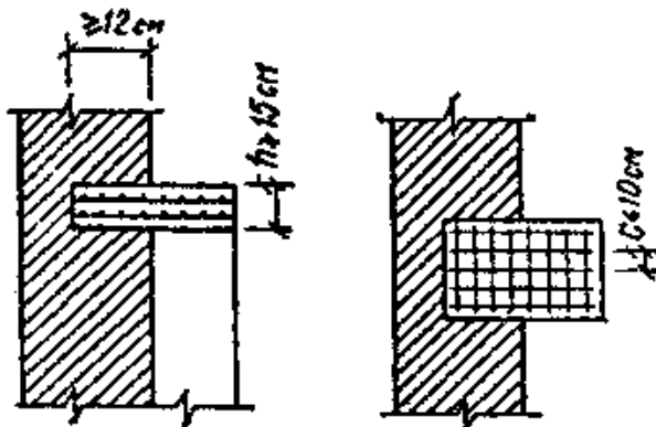
Рис. 13. Железобетонные распределительные плиты
