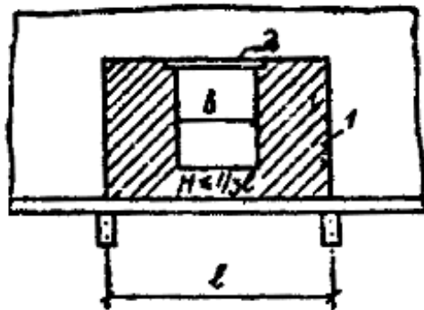
Рис. 17. Схема нагрузки на рандбалку при наличии проема в стене 1 - нагрузка на рандбалку, 2 - железобетонная перемычка
