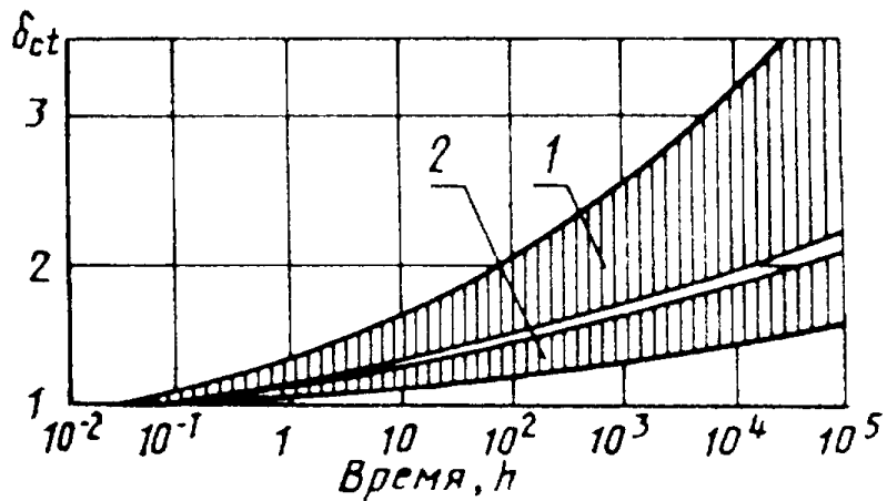
Коэффициенты ползучести при постоянном напряжении
