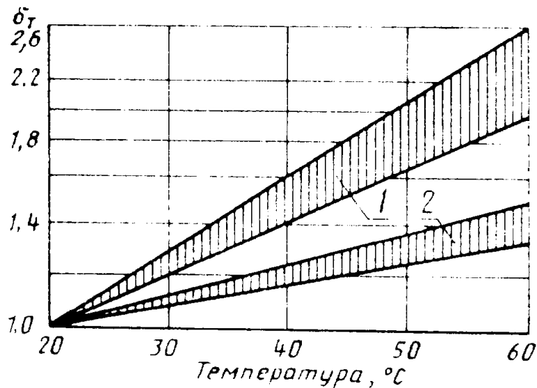
Коэффициенты температуры при постоянно действующих повышенных температурах
